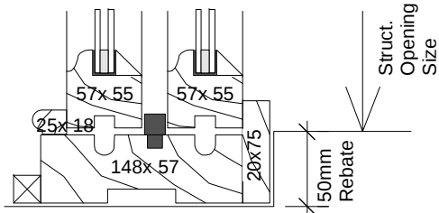
4. Jamb Detail
