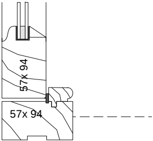
8. Jamb Detail
