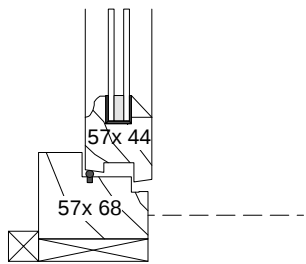
14. Jamb Detail
