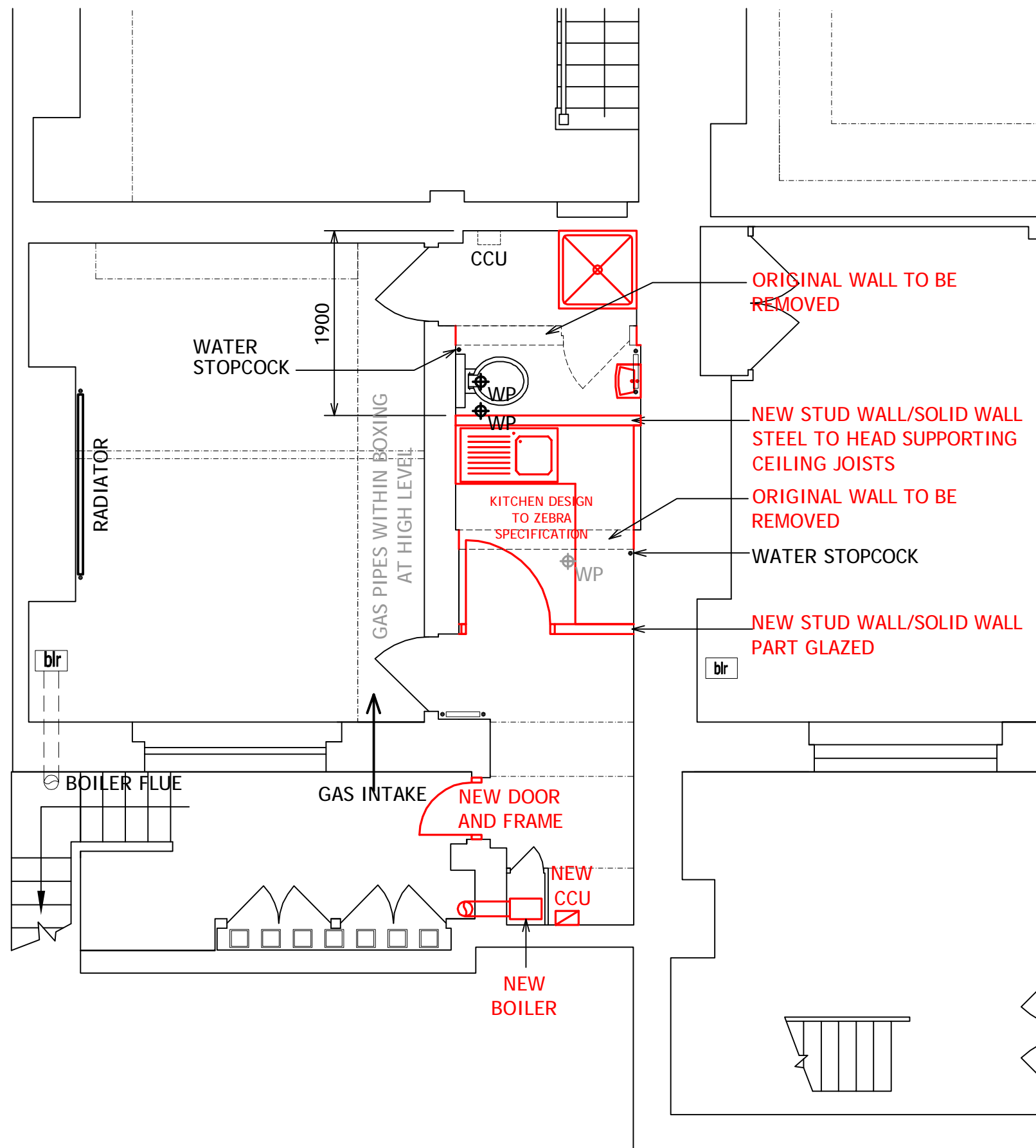
OPTION 1- 1:50
