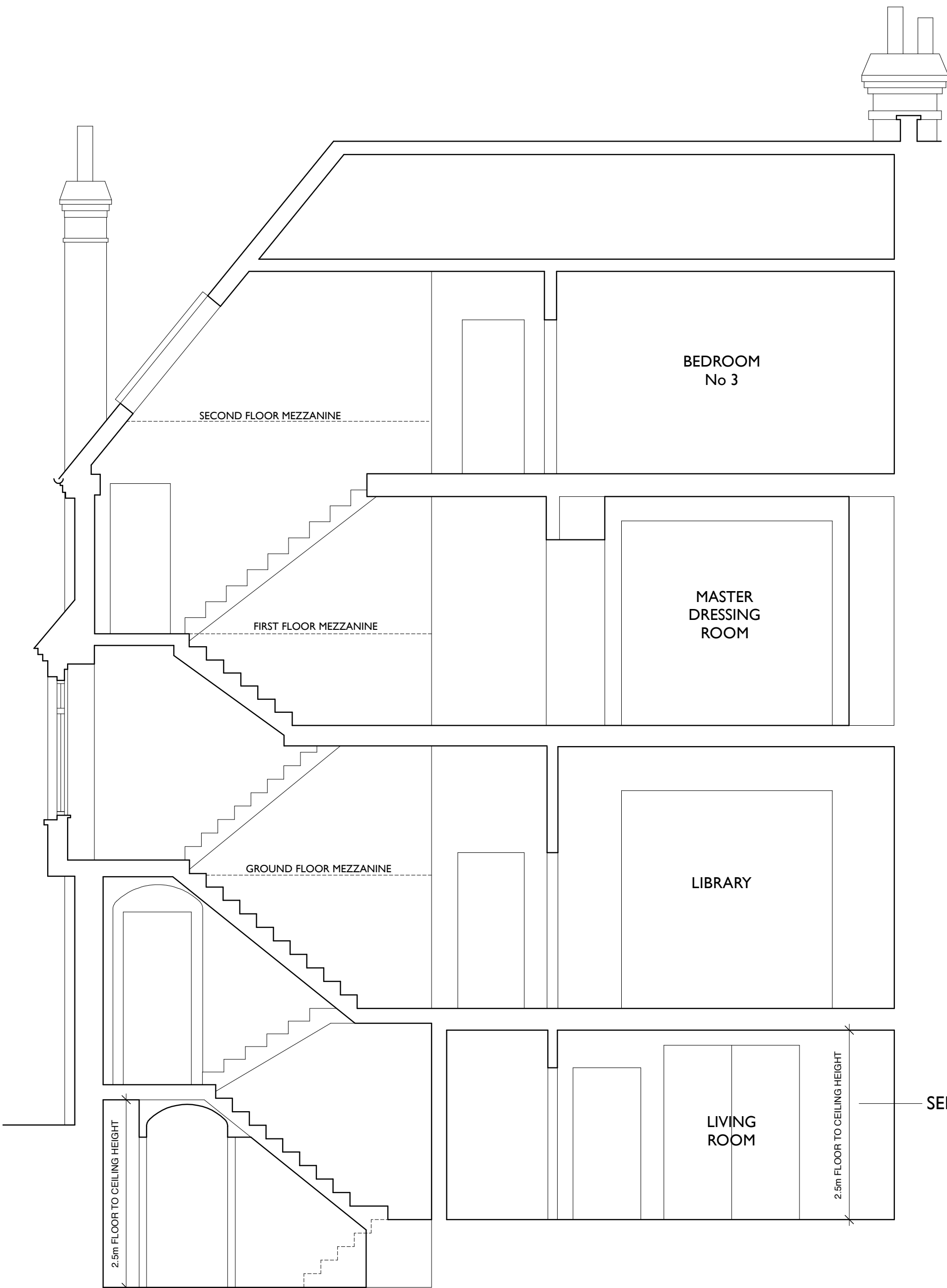
SECTION A-A
