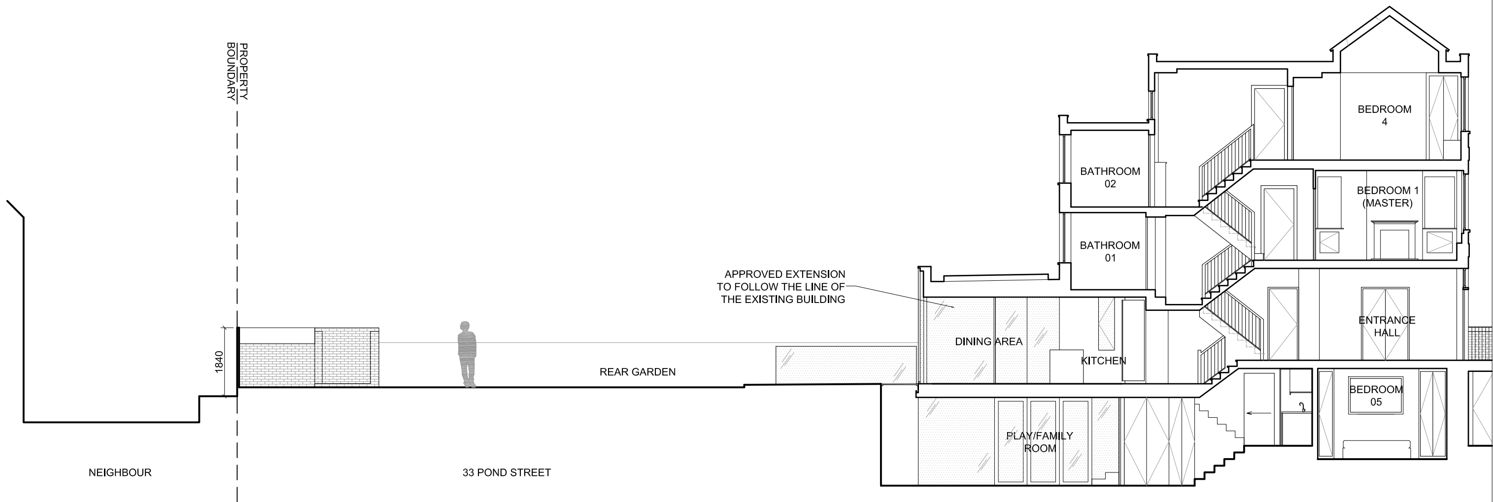
EXISTING SECTION A-A SCLAE 1:100
