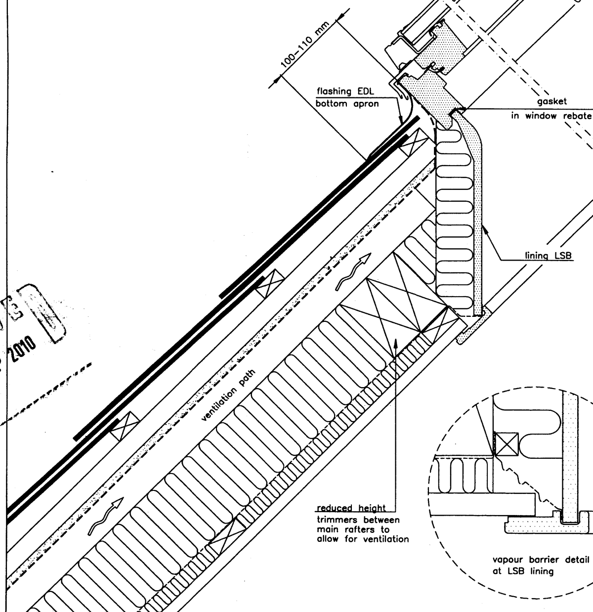
SECTION A-A 1:5
