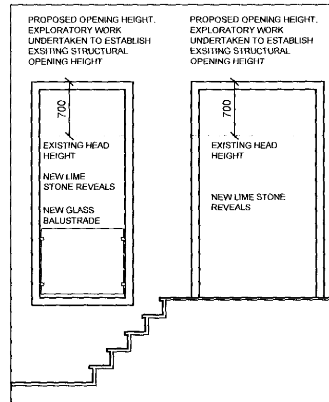
ELEVATION A
