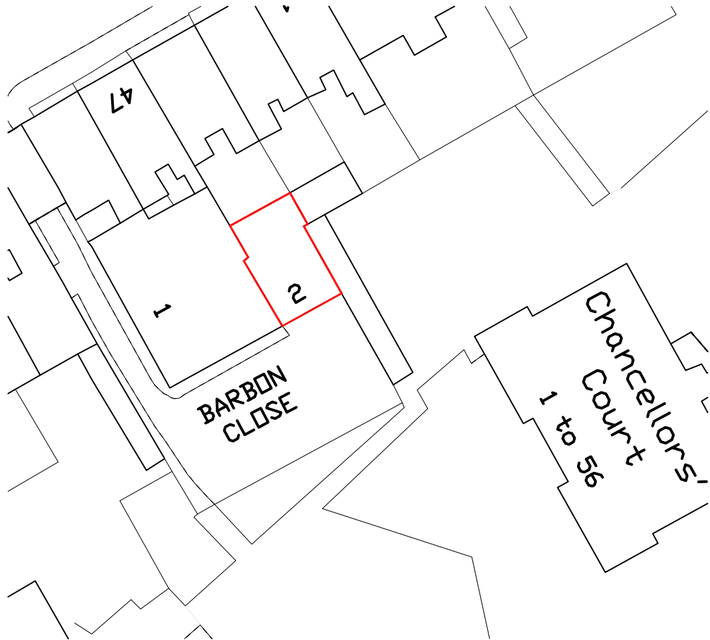
SITE PLAN 1:500
