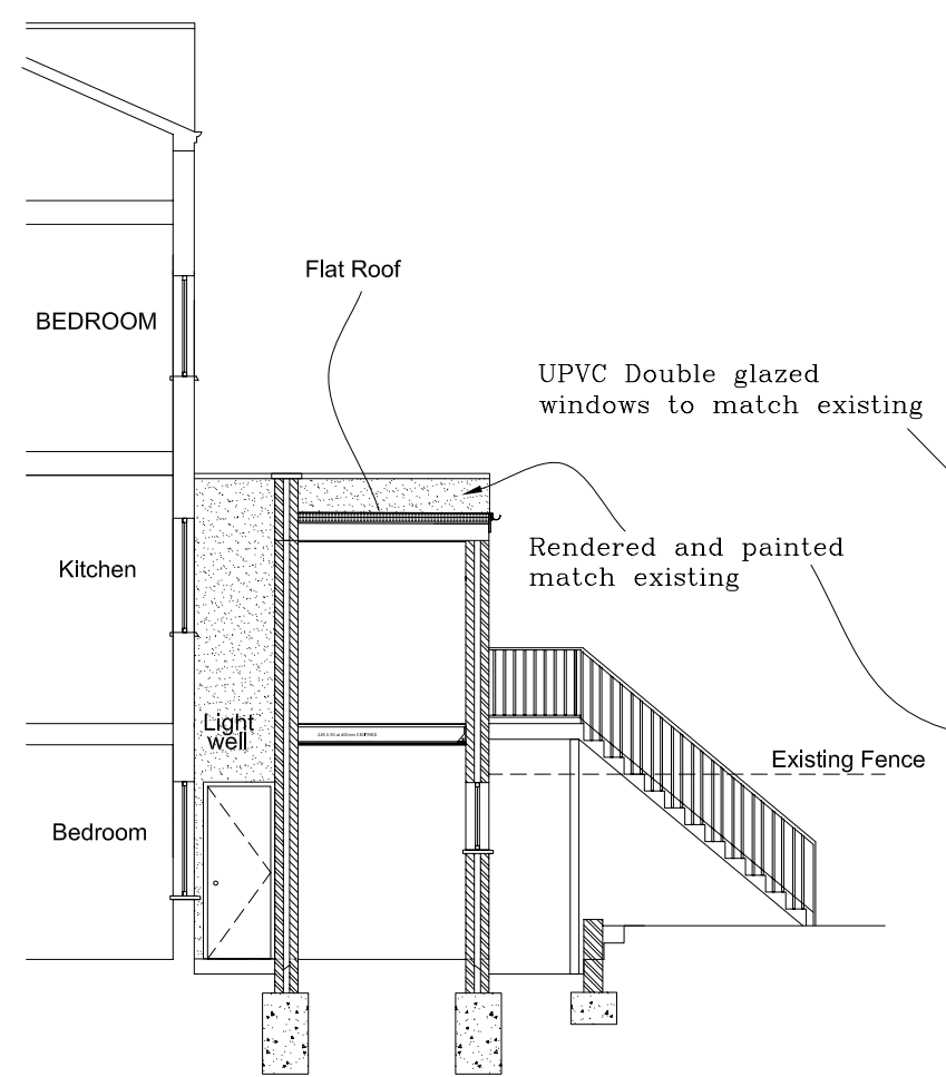
SECTION A-A 1:100
