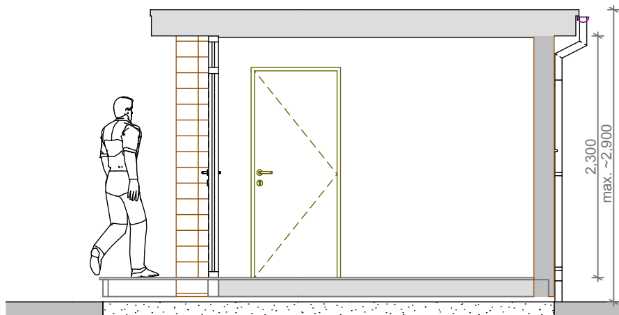
Section A-A: 1:50
