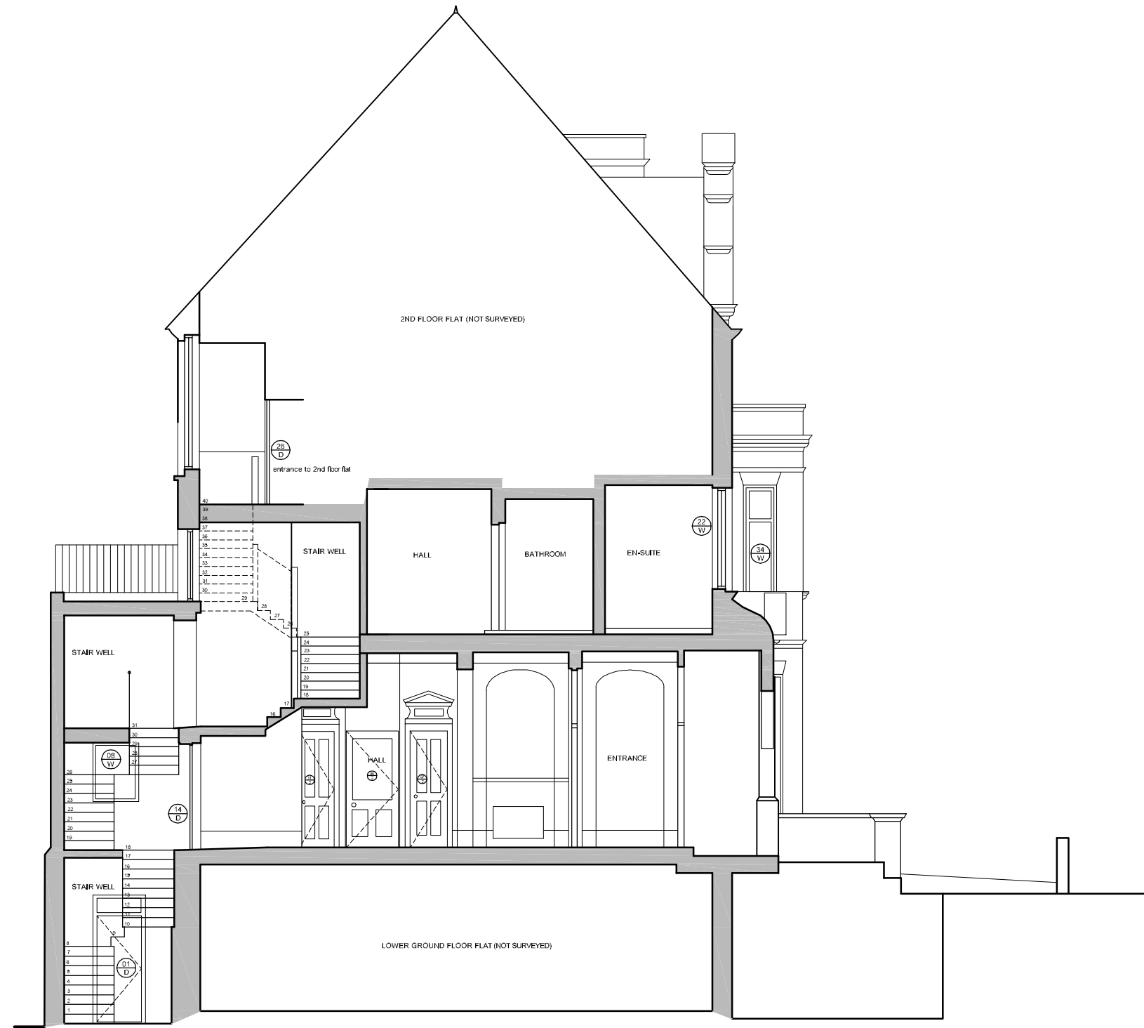
EXISTING SECTION DD
