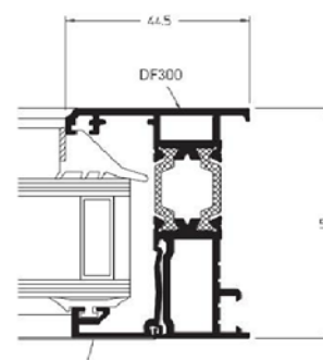
C Fixed Light Jamb
