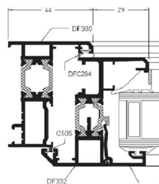
A Jamb / Vent
