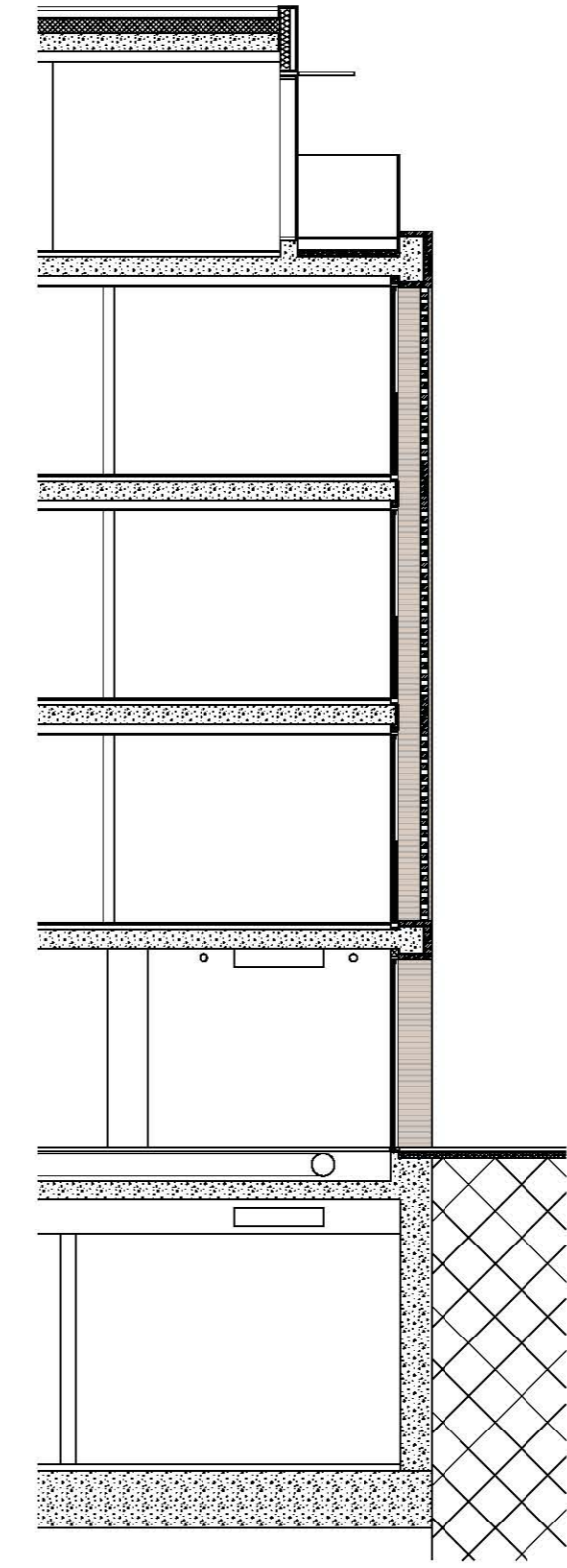
02 Section 1:50
