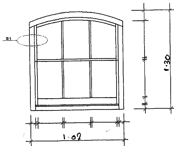
ELEVATION
