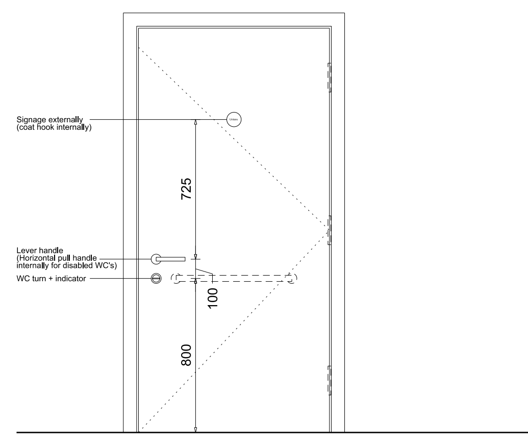
05 Typical toilet door
