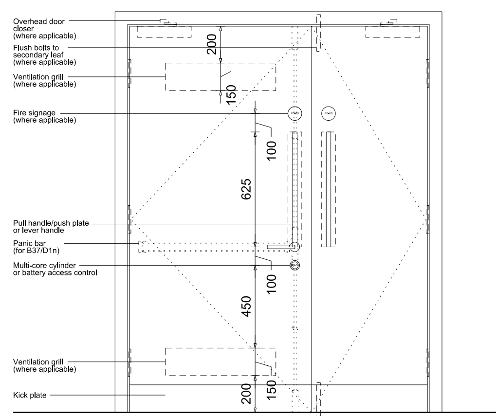
03 Basement Type T-2A
