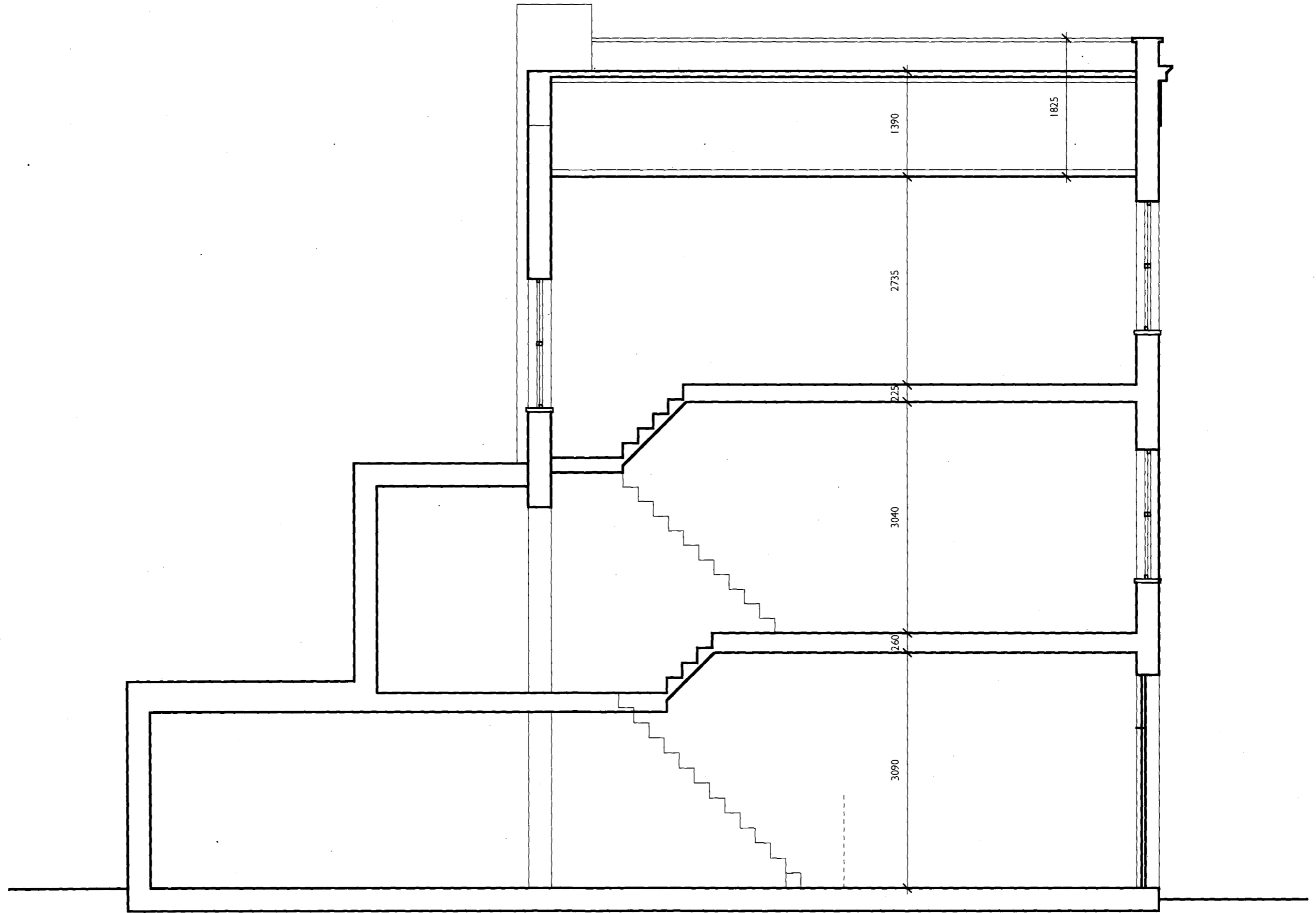
Existing Longitudinal Section
