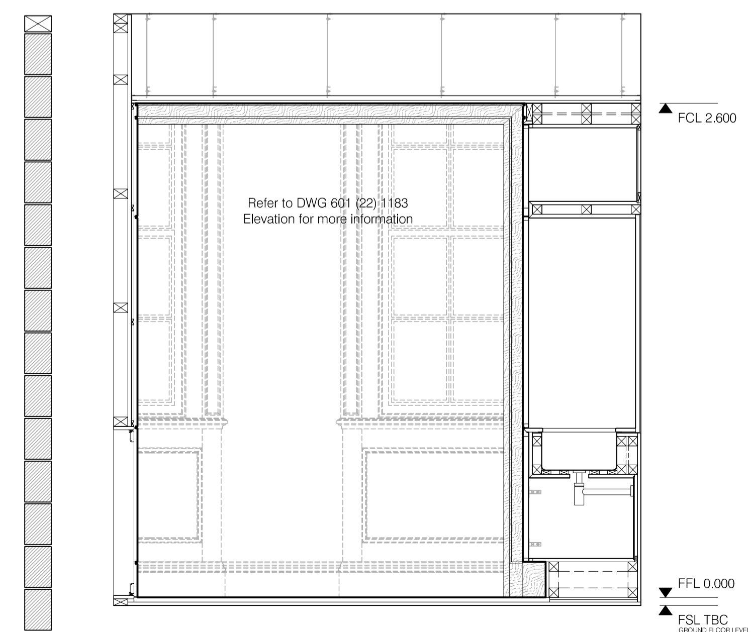
G18A SURVERY ELEVATION G Scale: 1:20 @ A1
