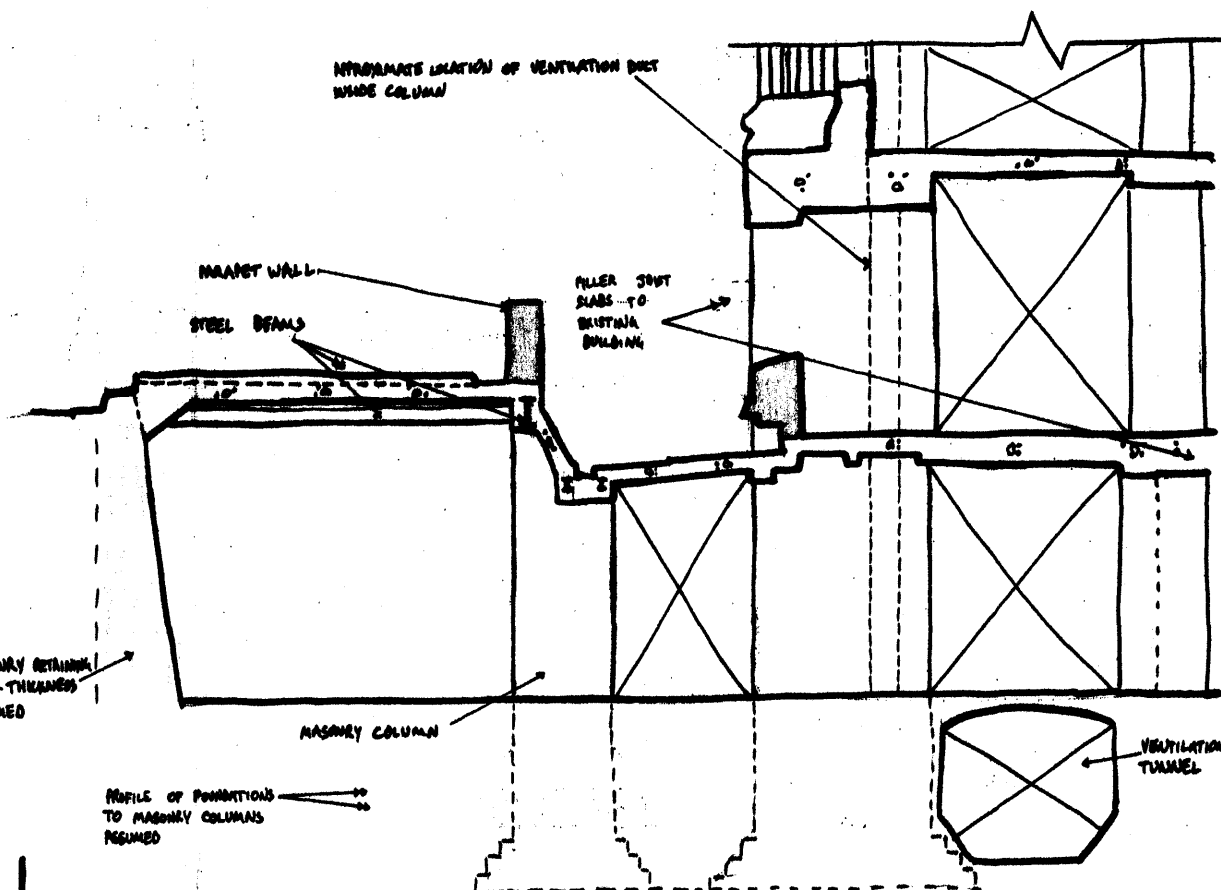
SECTION A-A
