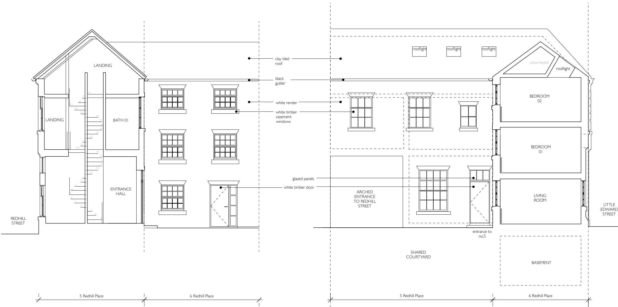
1 Elevation 01 Scale: 1:100
