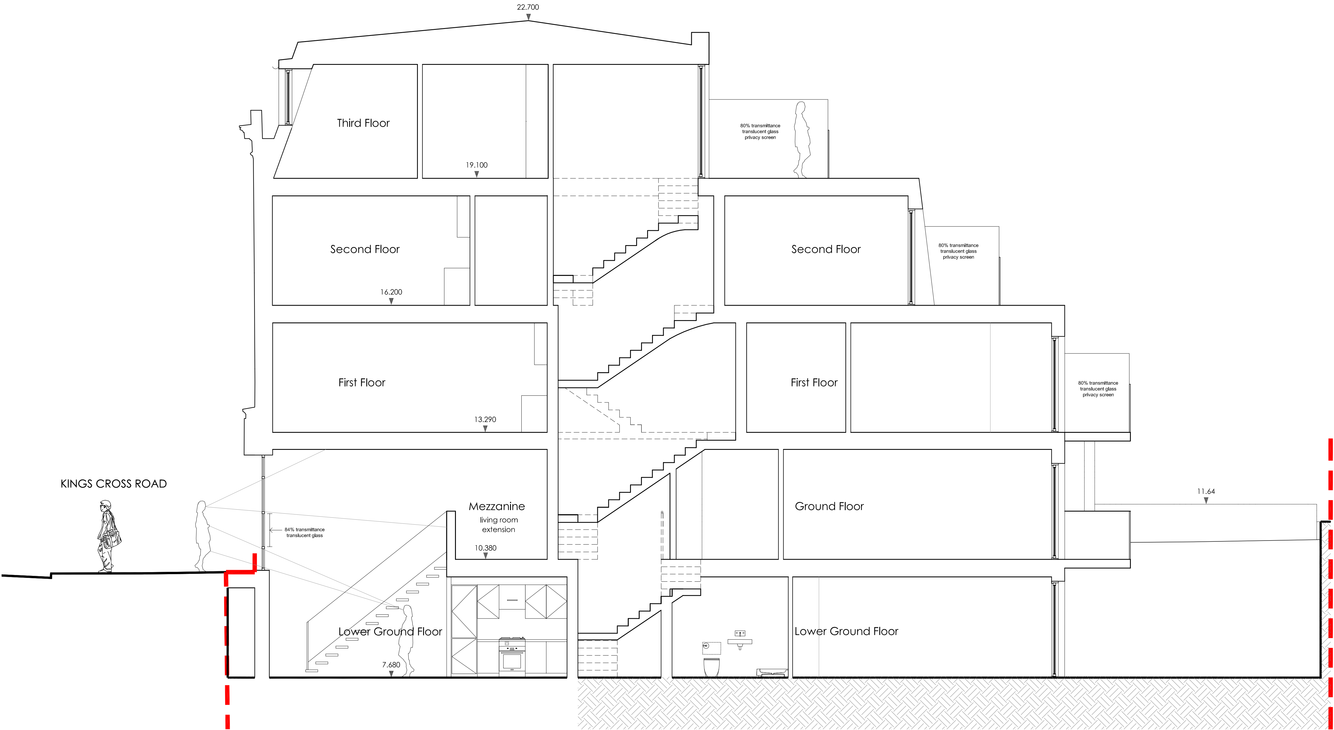
1 Section A-A
