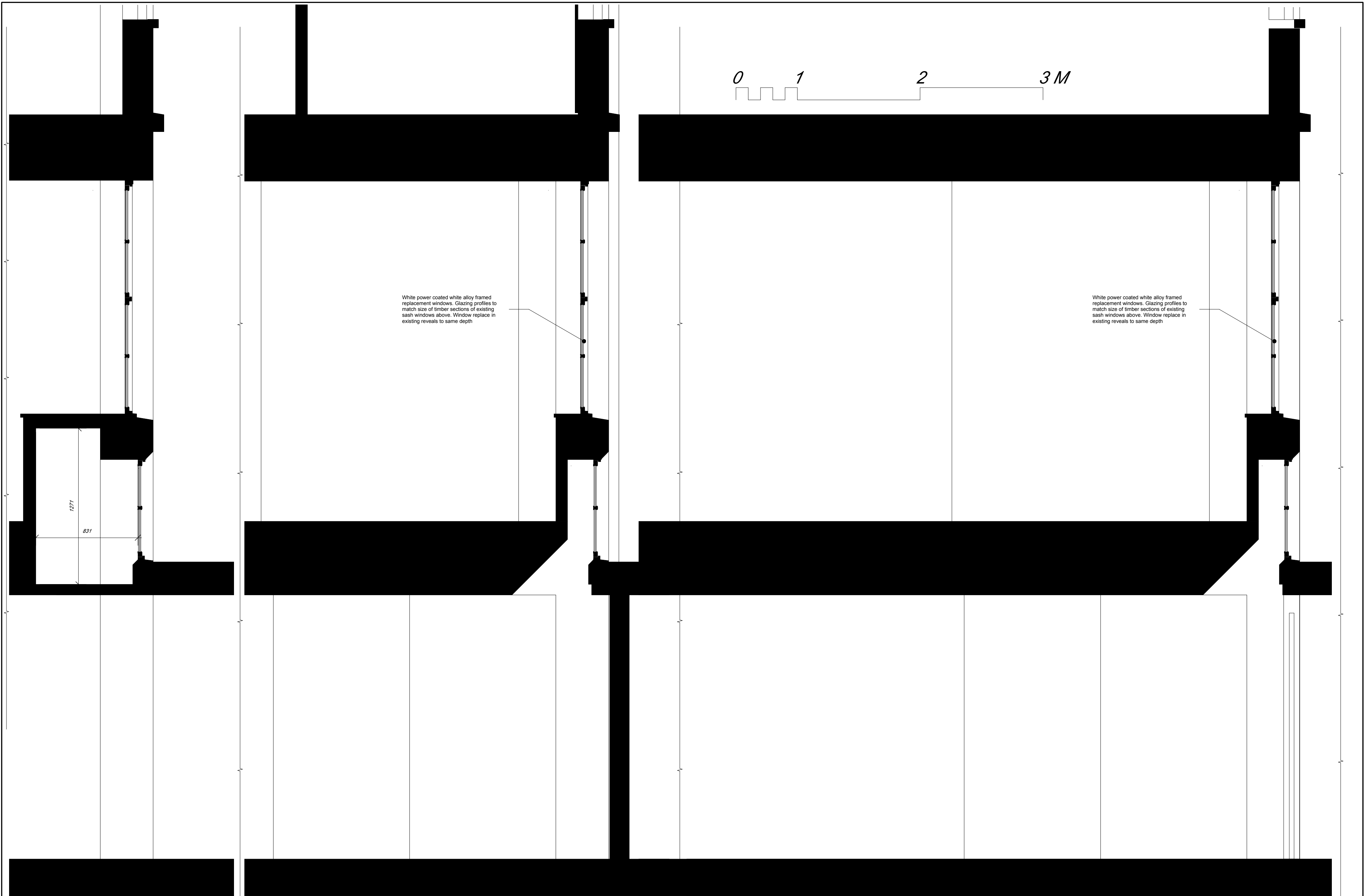
SECTION X - X scale: 1:20 SECTION Y - Y scale: 1:20 SECTION Z - Z scale: 1:20
