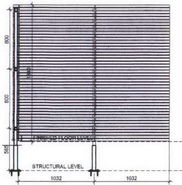
ELEVATION A
