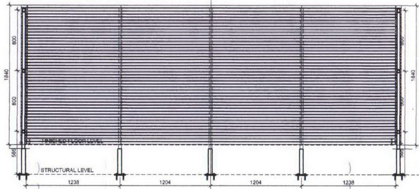
ELEVATION B
