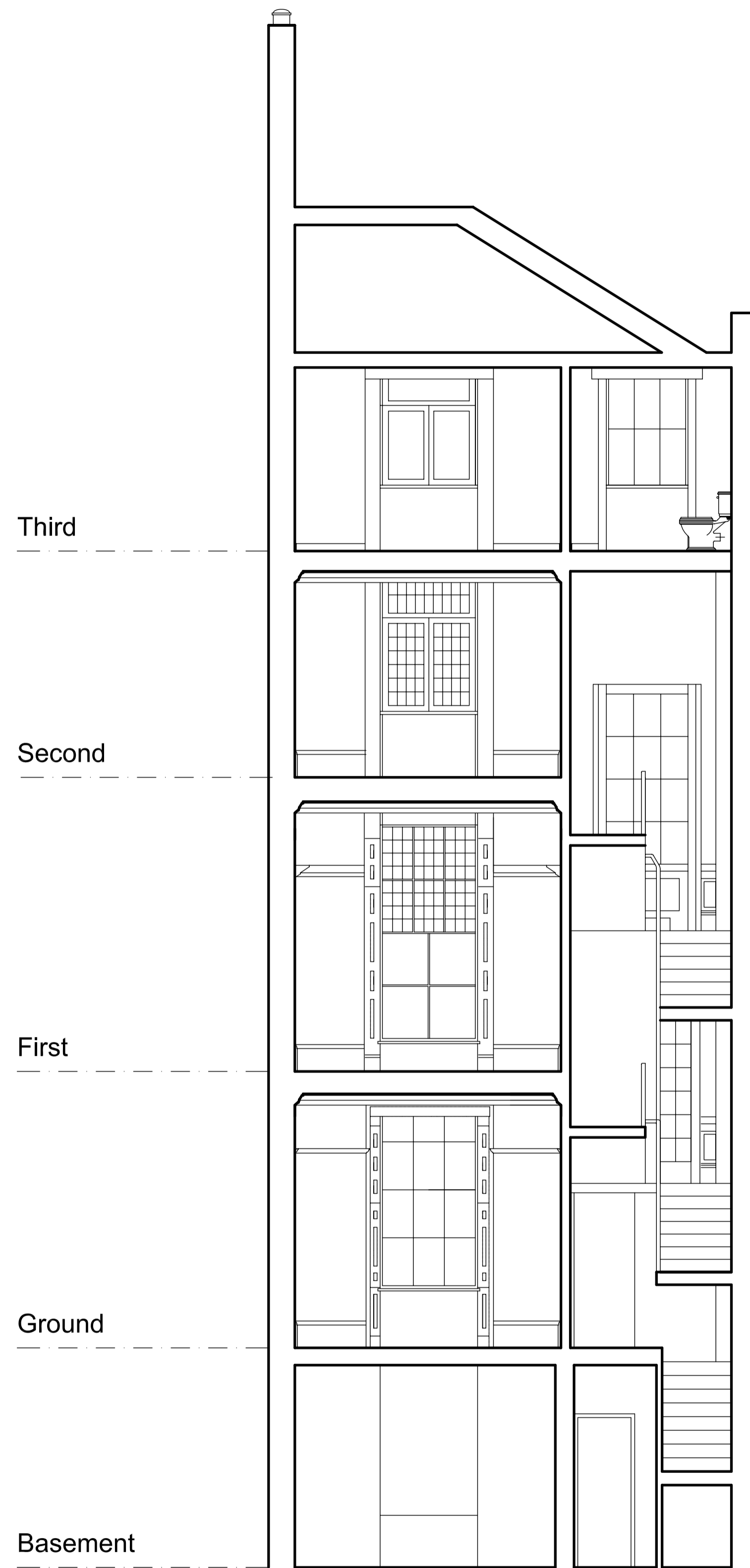
Section DD
