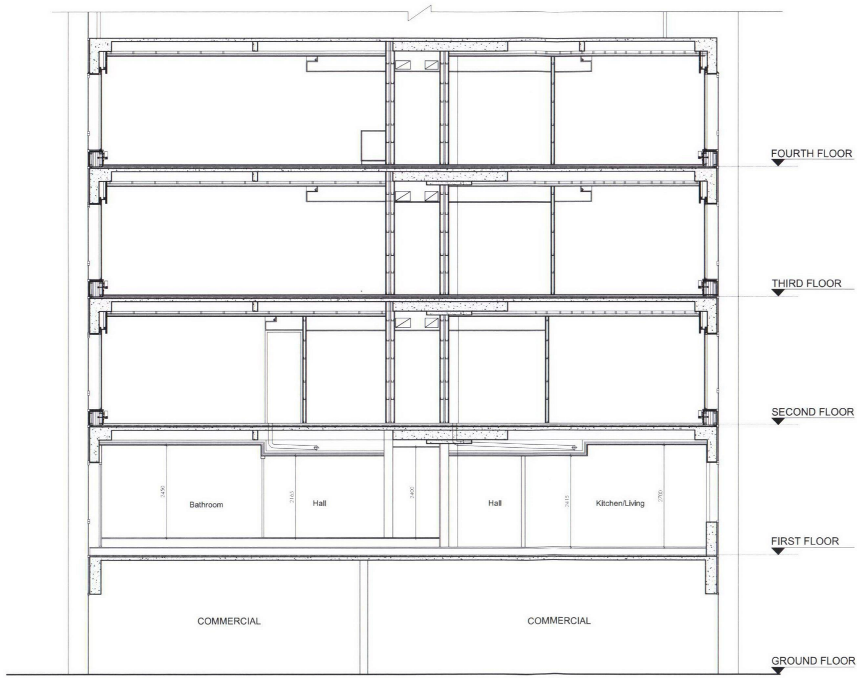
SECTION A-A
