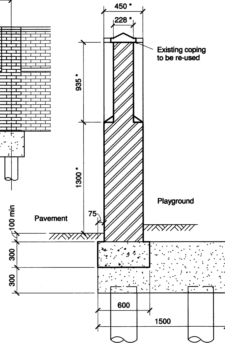
Section 1 1 : 25 XX-XX-0001
