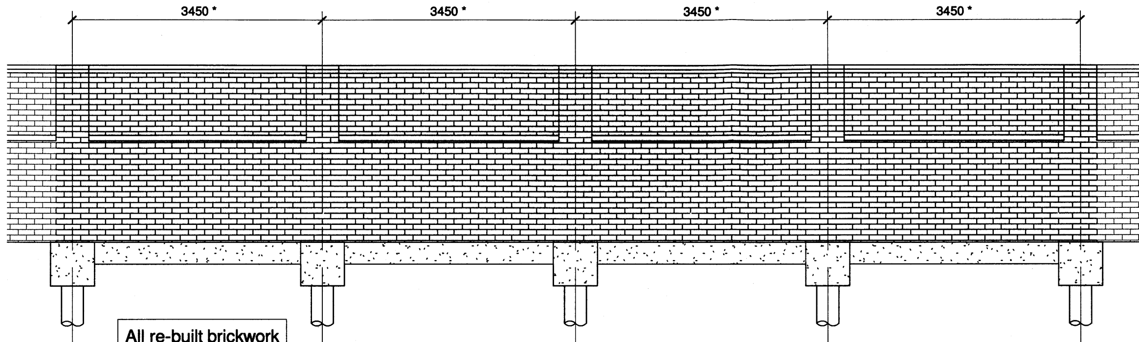
Section 2 1 : 50 XX-XX-0001
