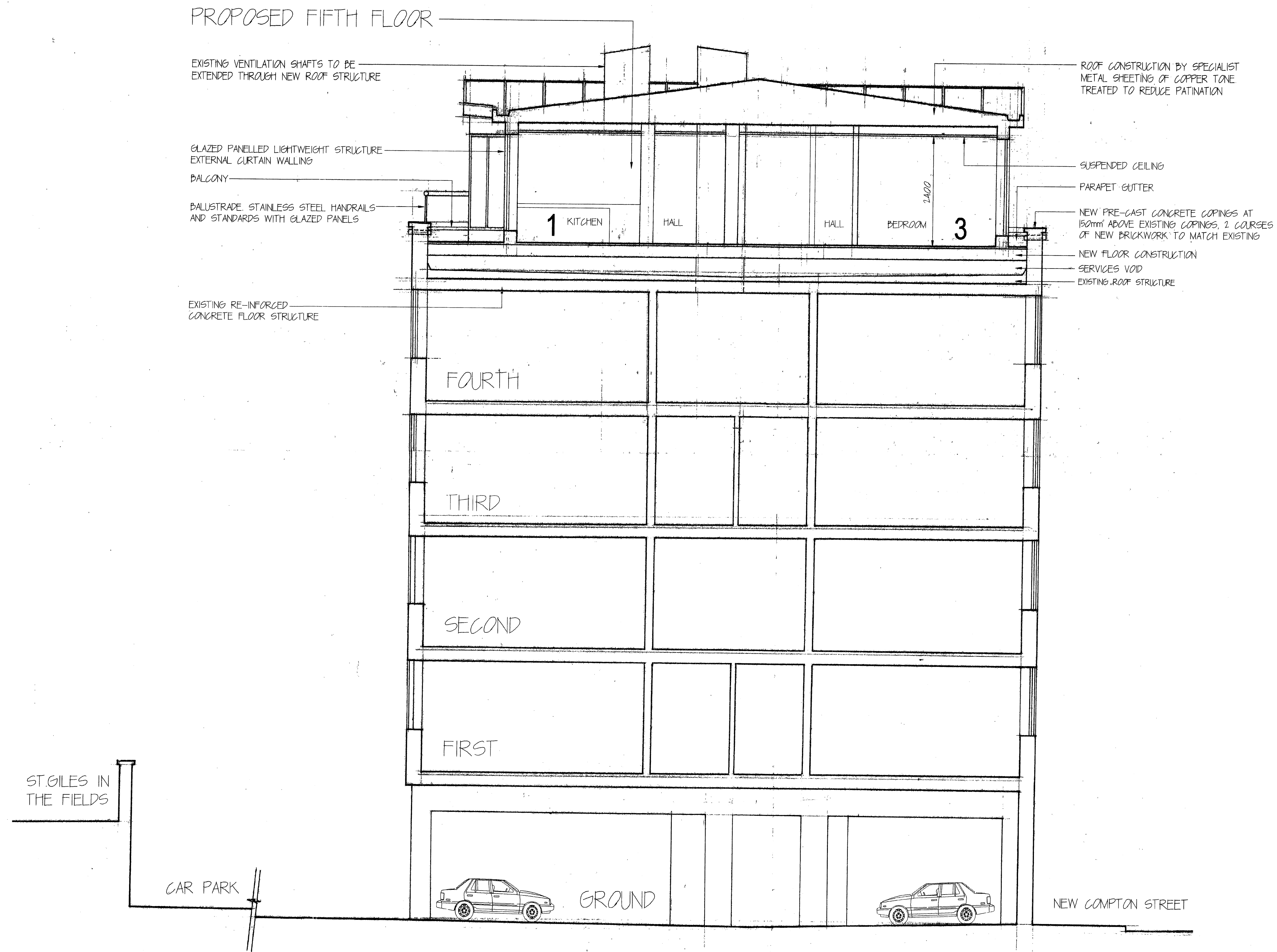
SECTION X-X (N.T.S.)
