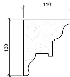
CORNICE TYPE - C1
