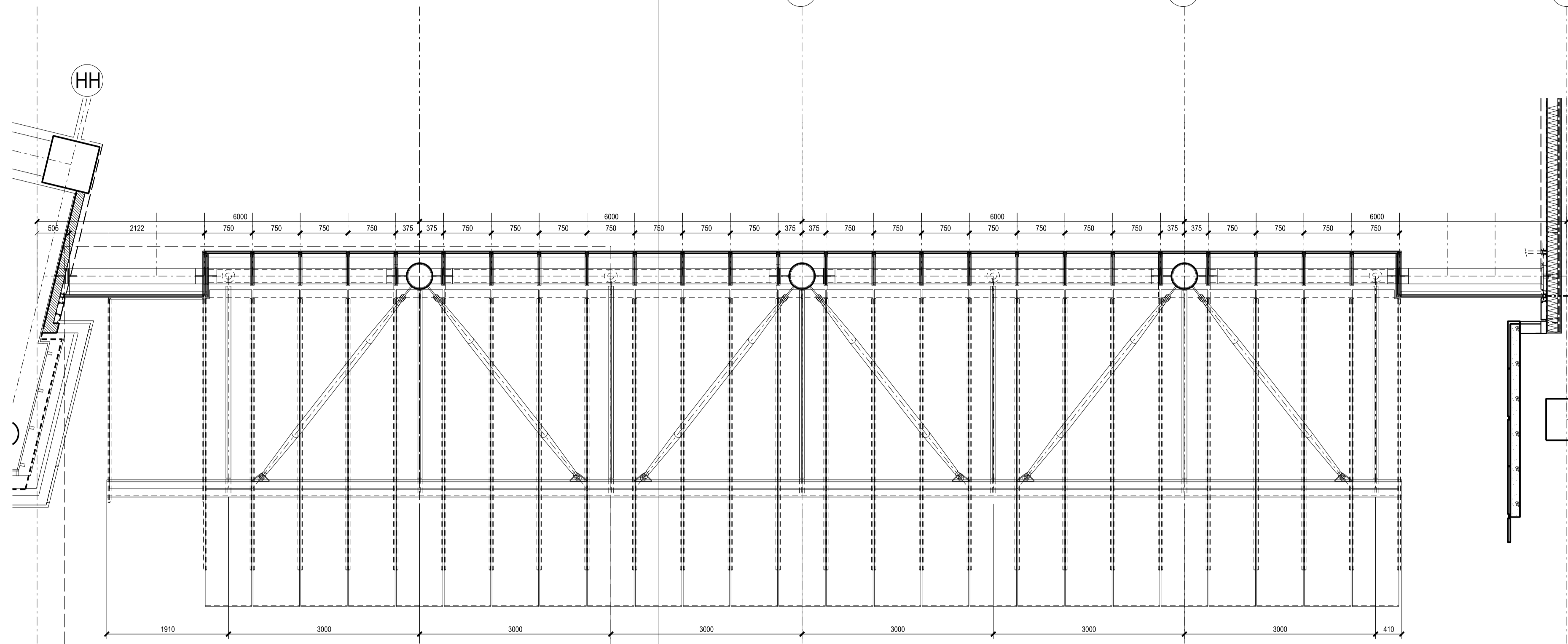
1 Plan 1:50
