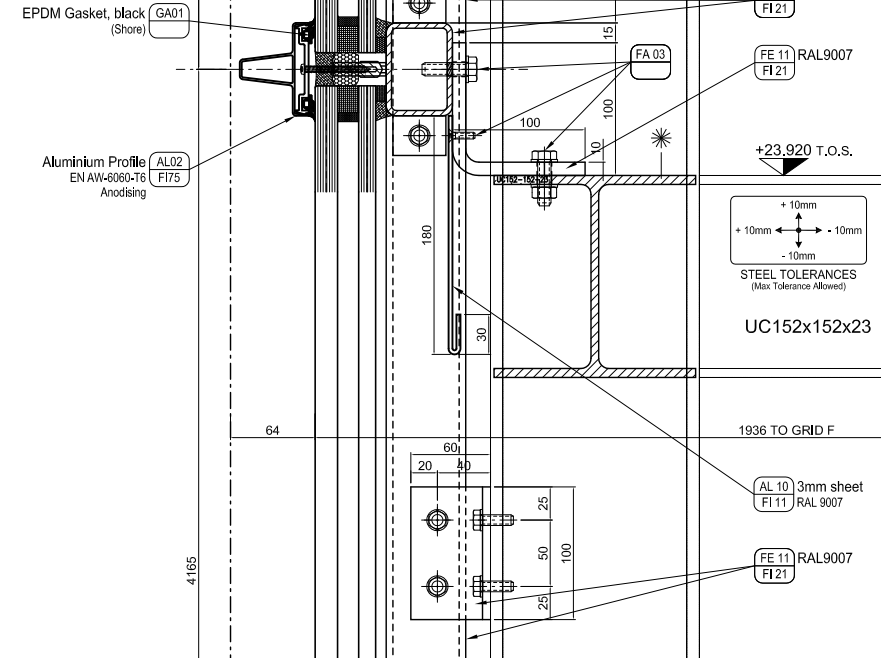
02 Vertical section Scale: 1:2
