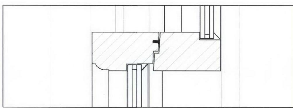
Transom
