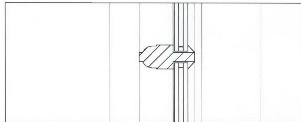
Glazing bar
