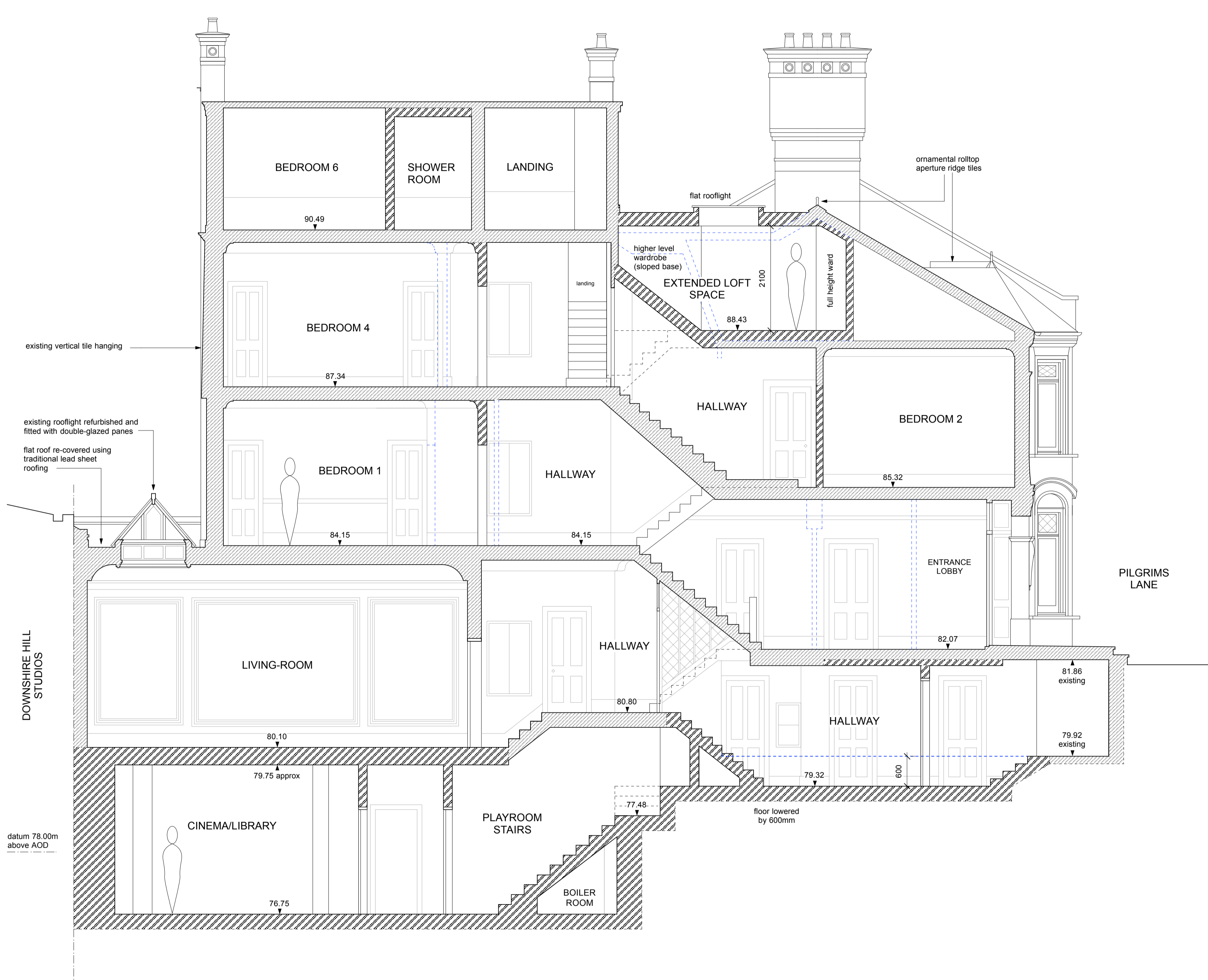
SECTION A-A
