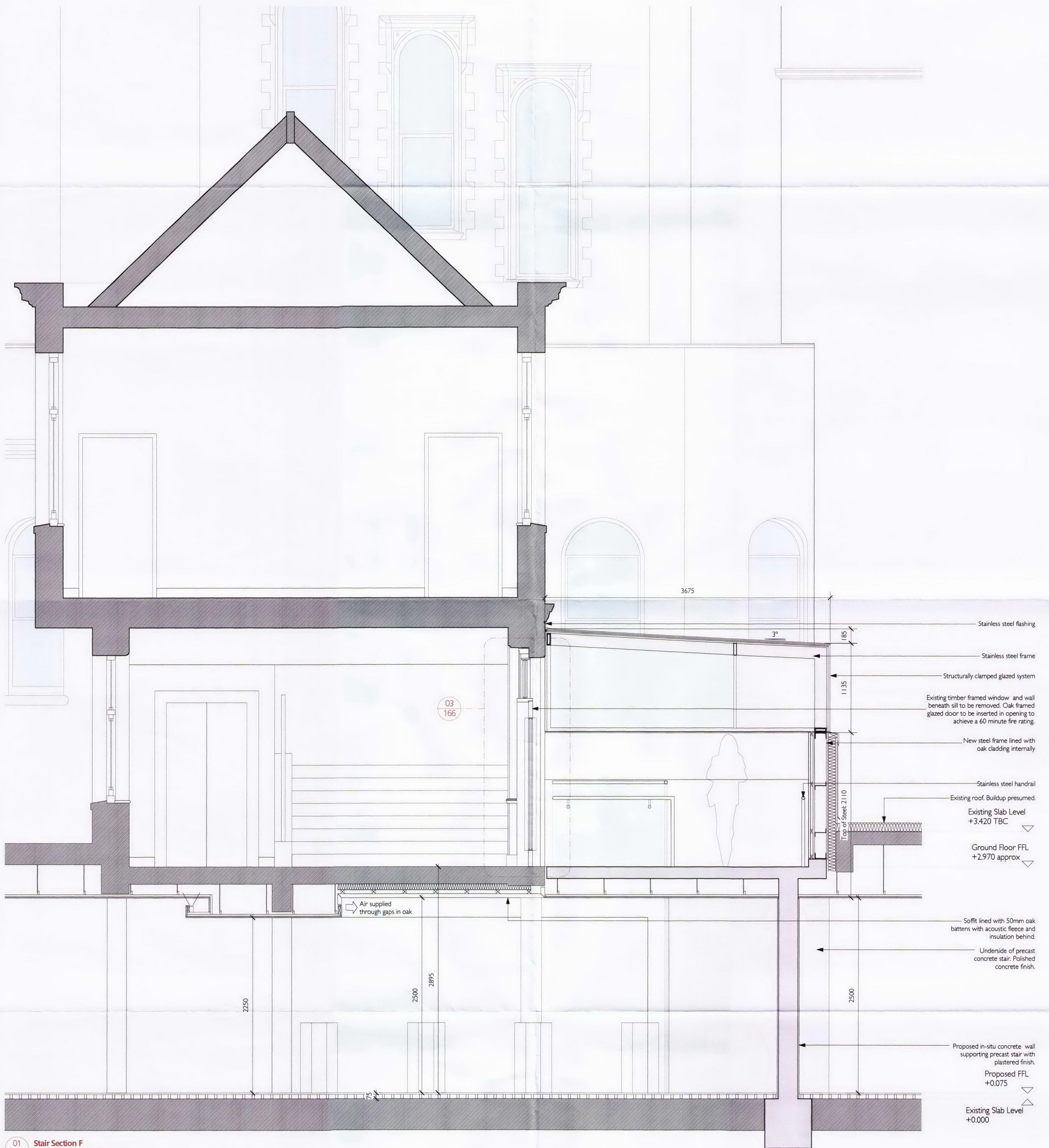
01 Stair Section F 1:25
