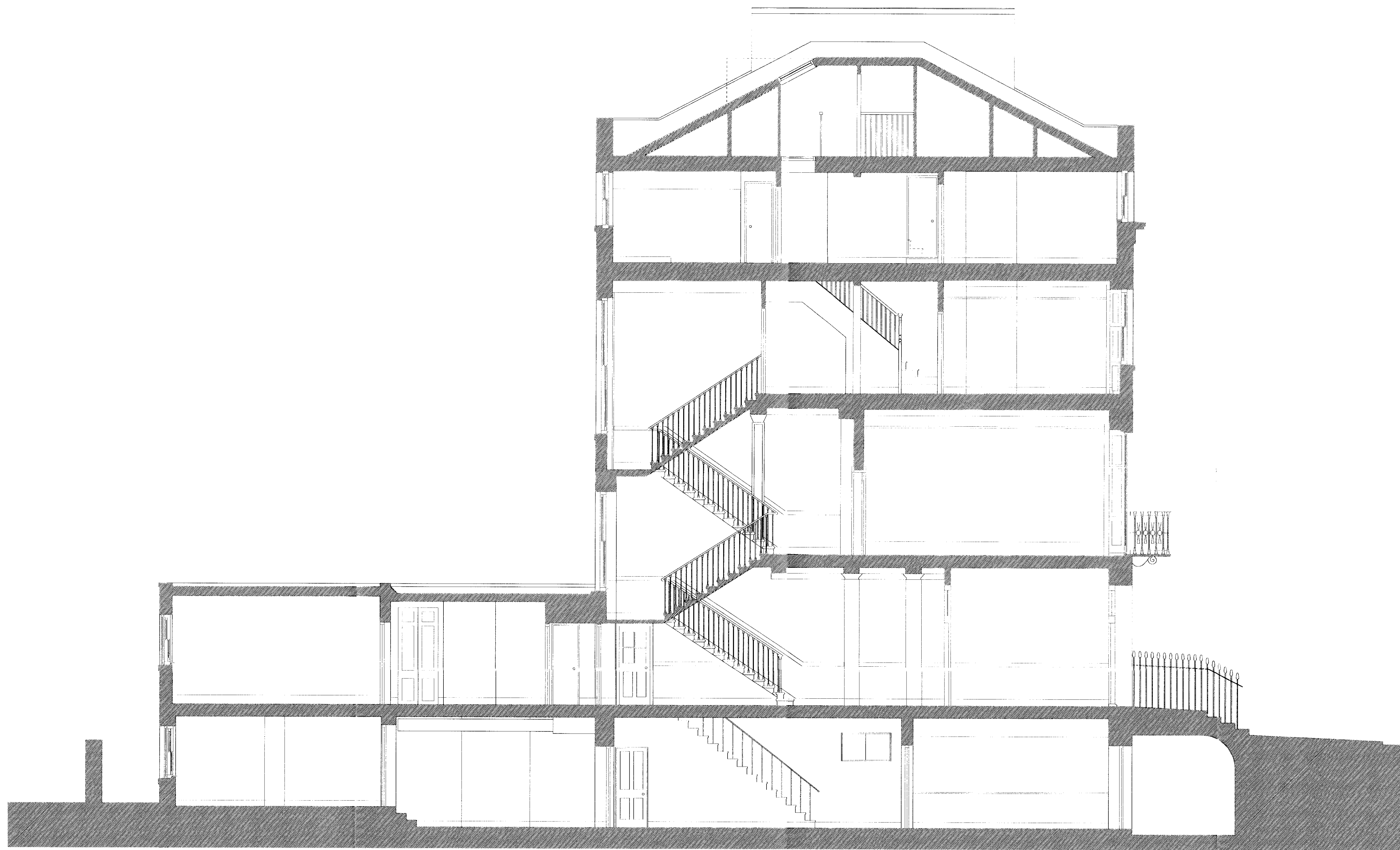
1 Existing Section AA 1:100 @ A3 & 1:50 @ A1
