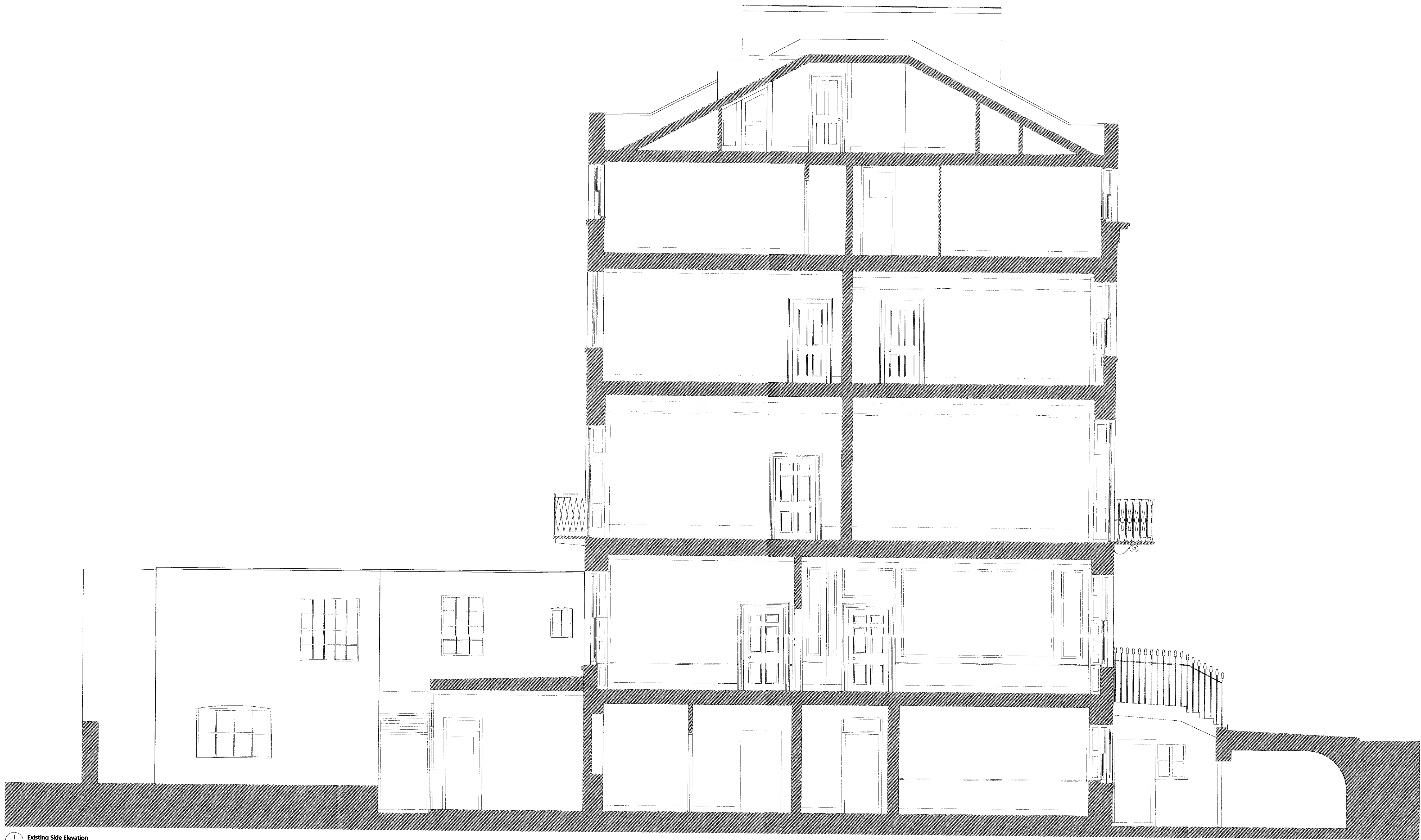
Existing Side Elevation 1:100 @ A3 & 1:50 @ A1
