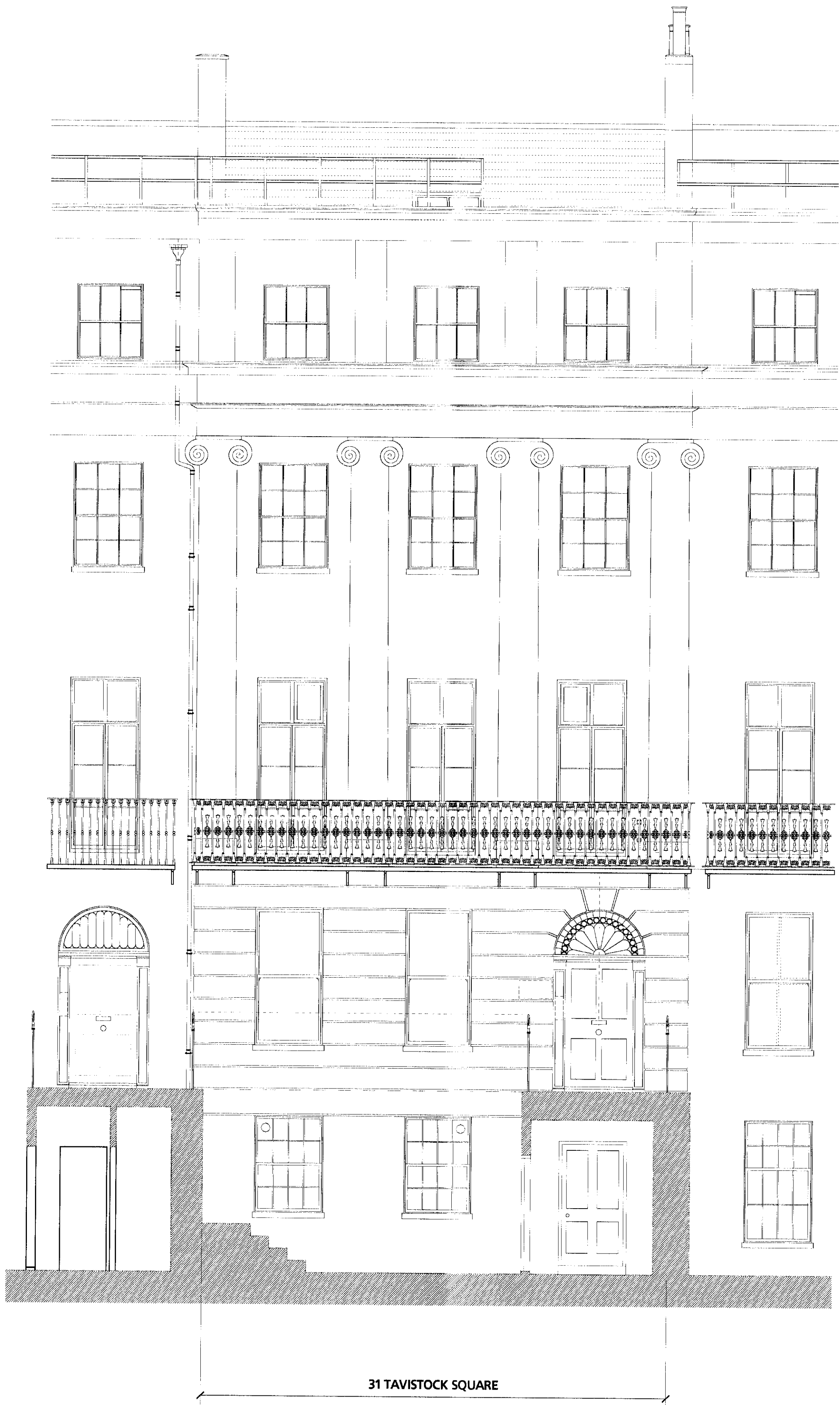
1 Existing Front Elevation 1:100 @ A3 & 1:50 @ A1
