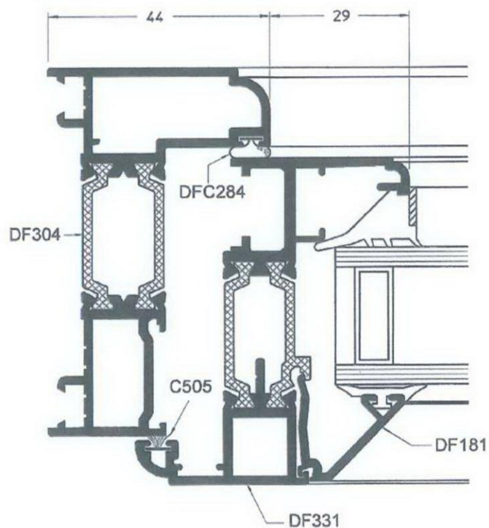
A Jamb / Vent
