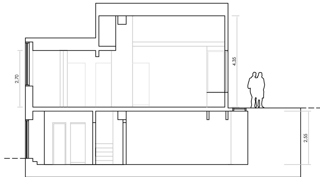
SECTION A-A
