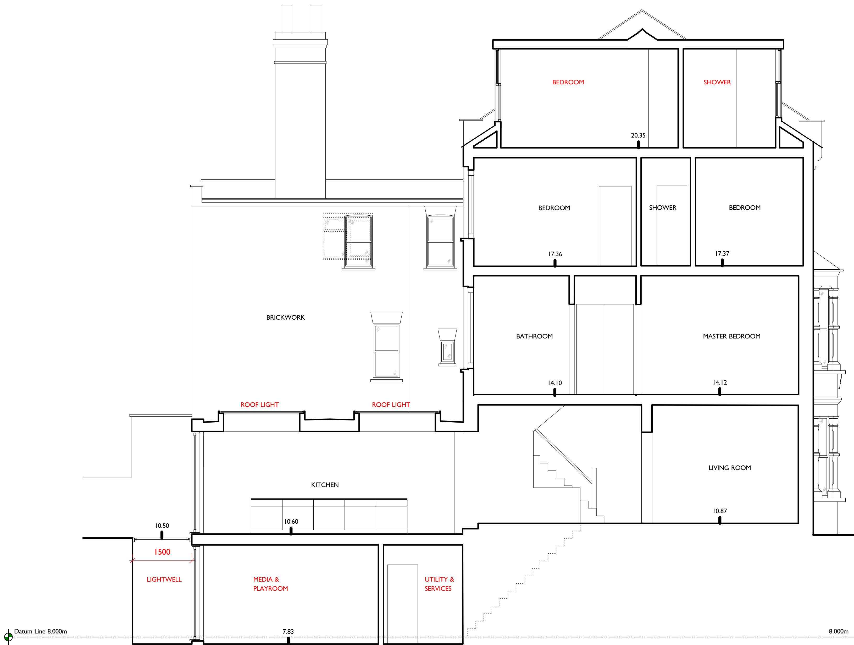
1 SECTION A-A Scale: 1:50
