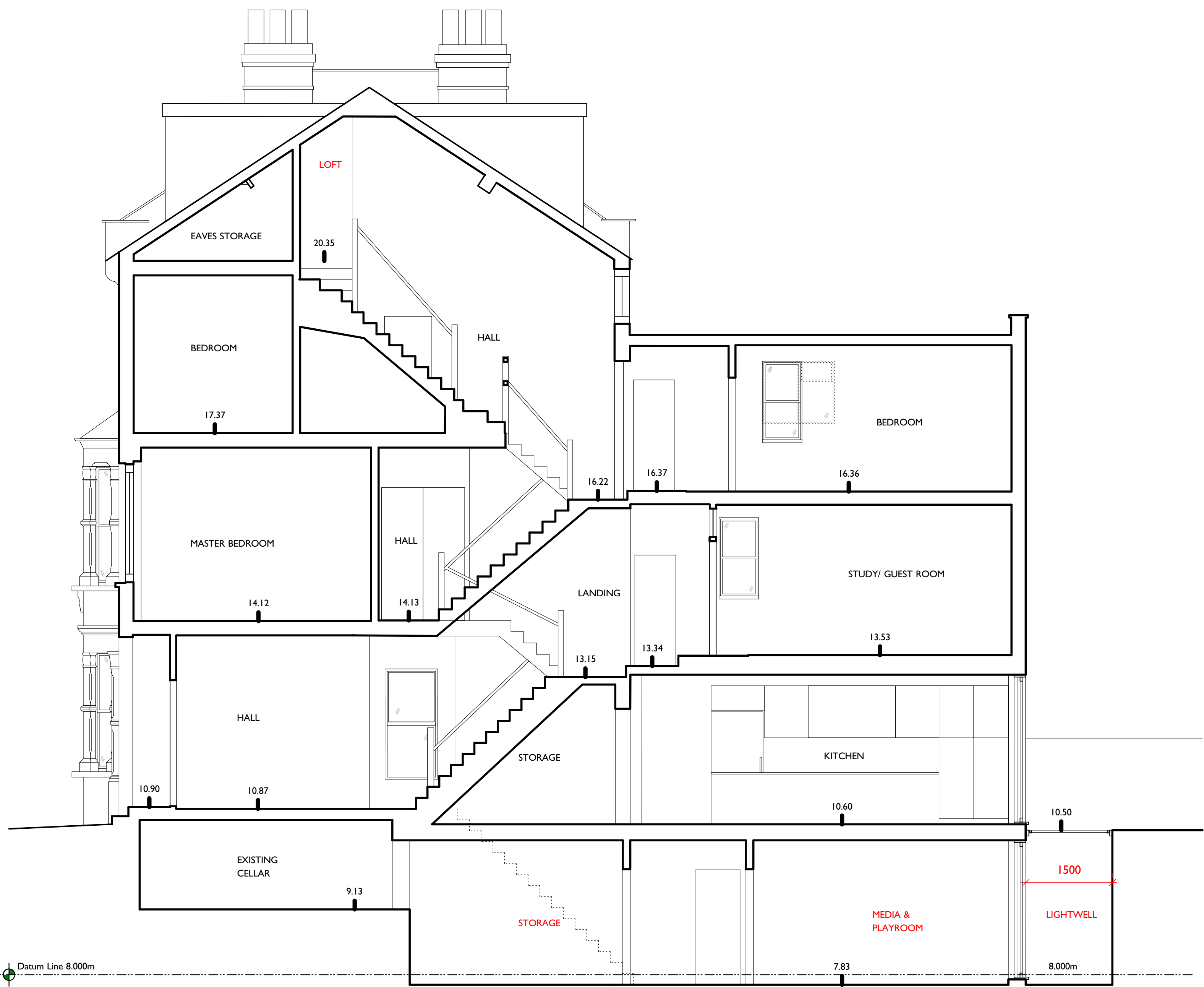
2 SECTION B-B Scale: 1:50
