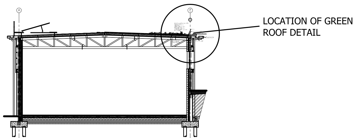
SECTION A-A 1:200
