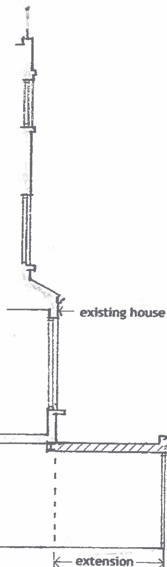
SECTION A-A
