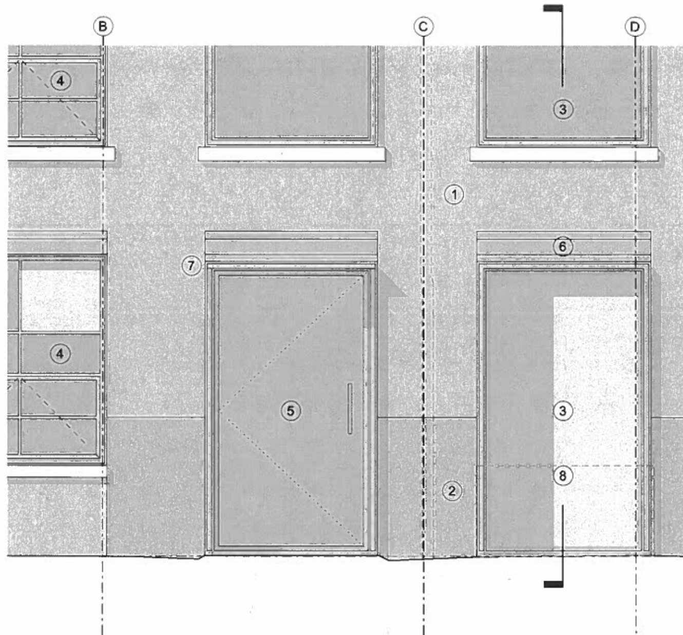
ELEVATION
