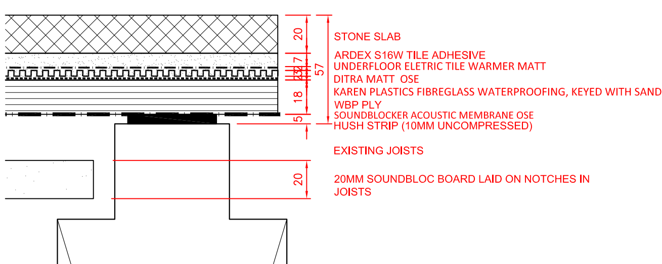
BATHROOM DETALS 1:2
