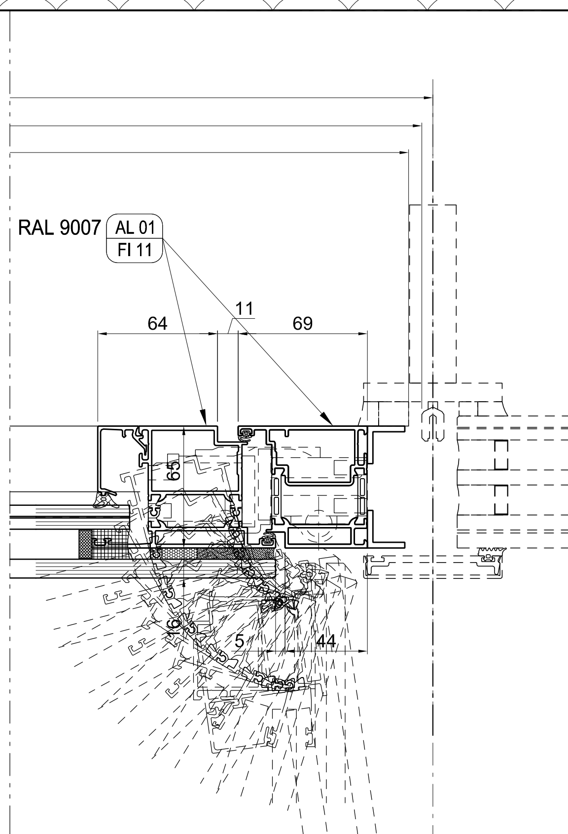
4 VERTICAL SECTION Door type 15 Scale: 1:2
