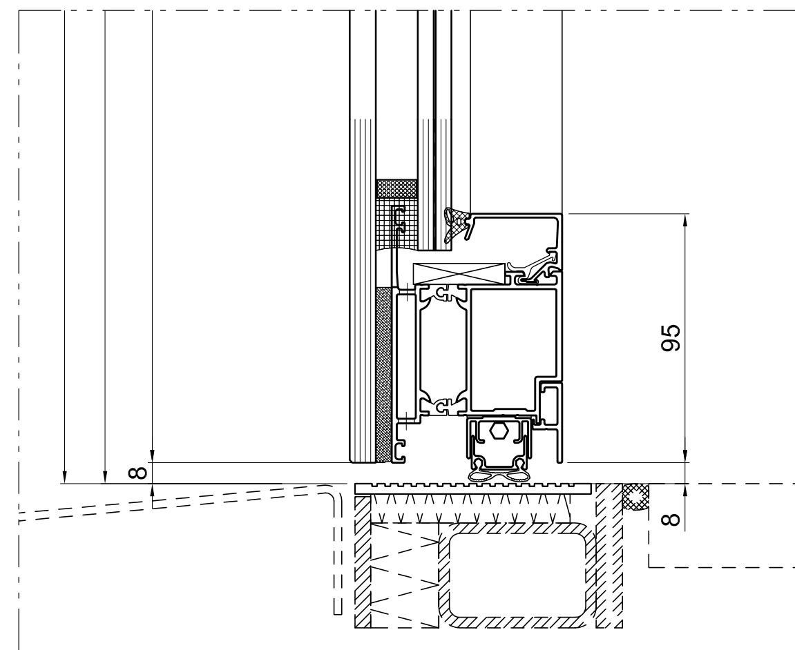
5 VERTICAL SECTION Door type 15 Scale: 1:2
