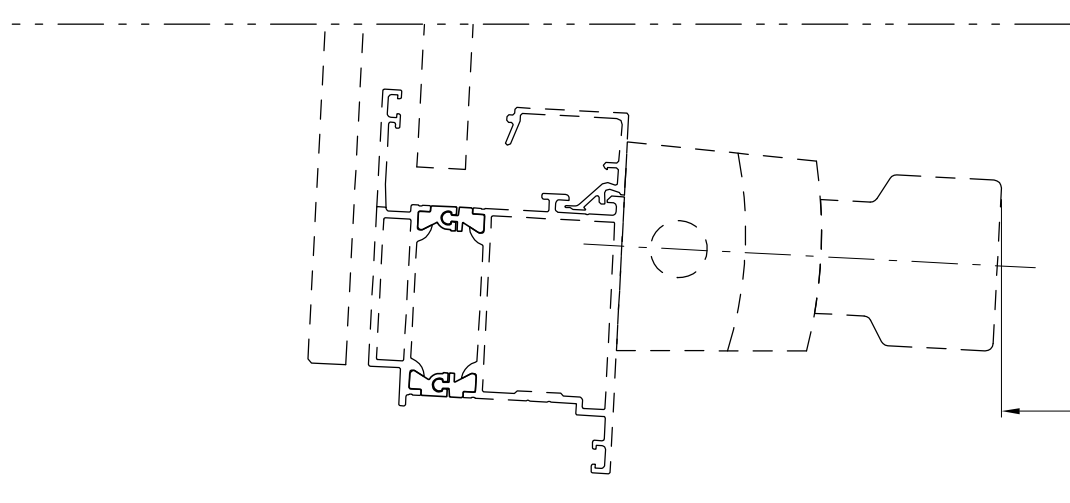
1 HORIZONTAL SECTION Door type 15 Double Scale: 1:2
