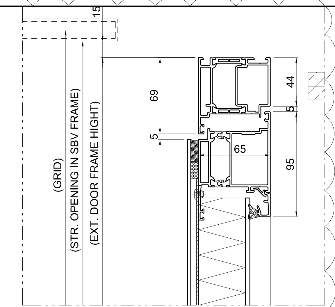
8 VERTICAL SECTION Door type 12 Scale: 1:2
