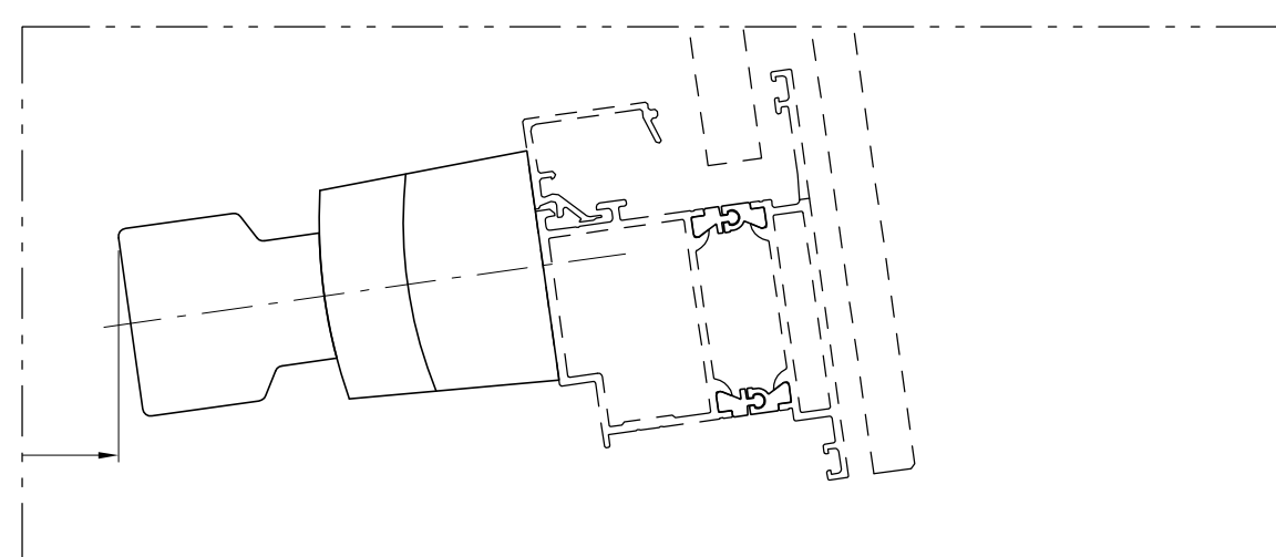
3 HORIZONTAL SECTION Door type 15 Double Scale: 1:2
