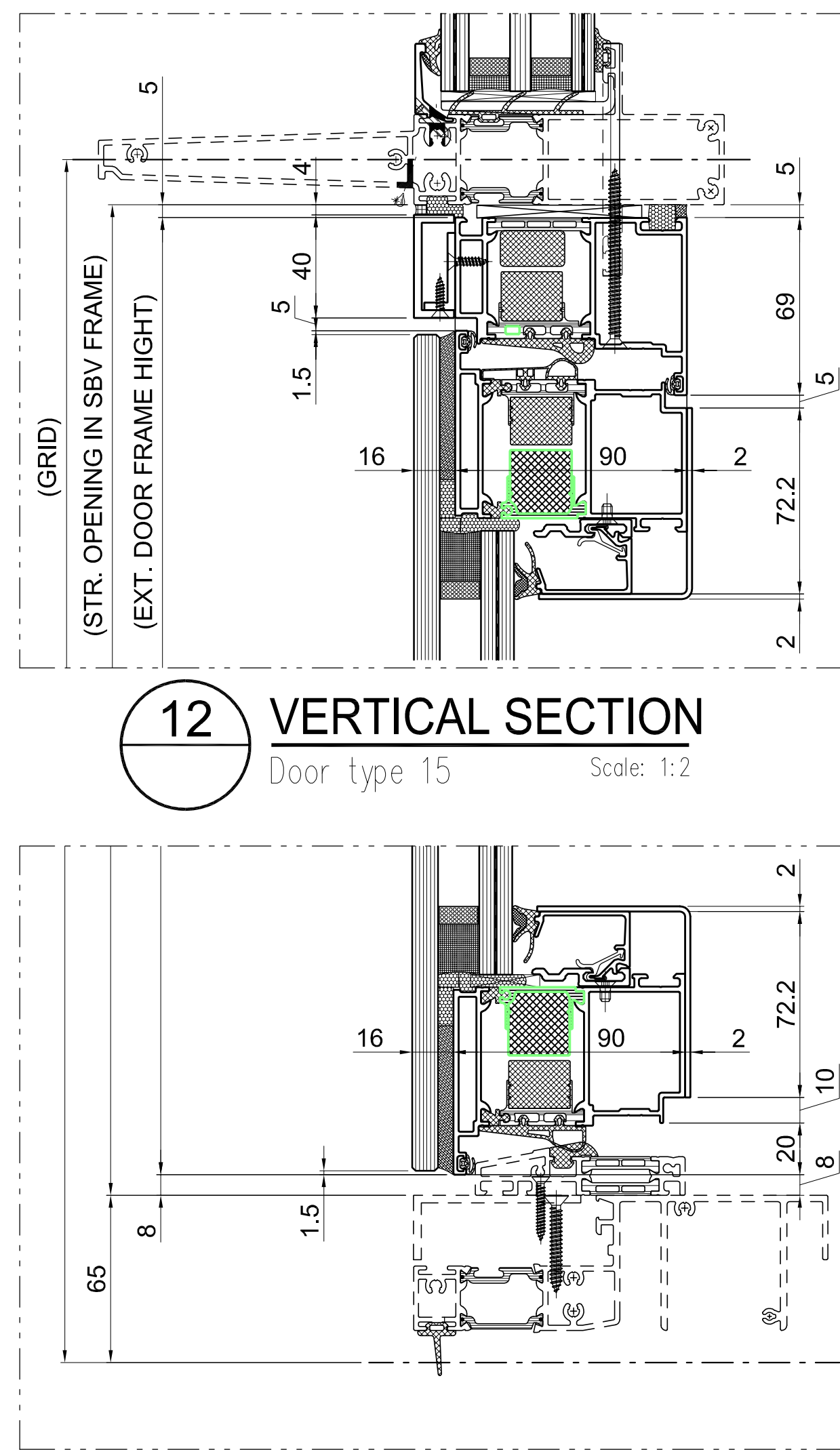
12 VERTICAL SECTION Door type 15 Scale: 1:2
