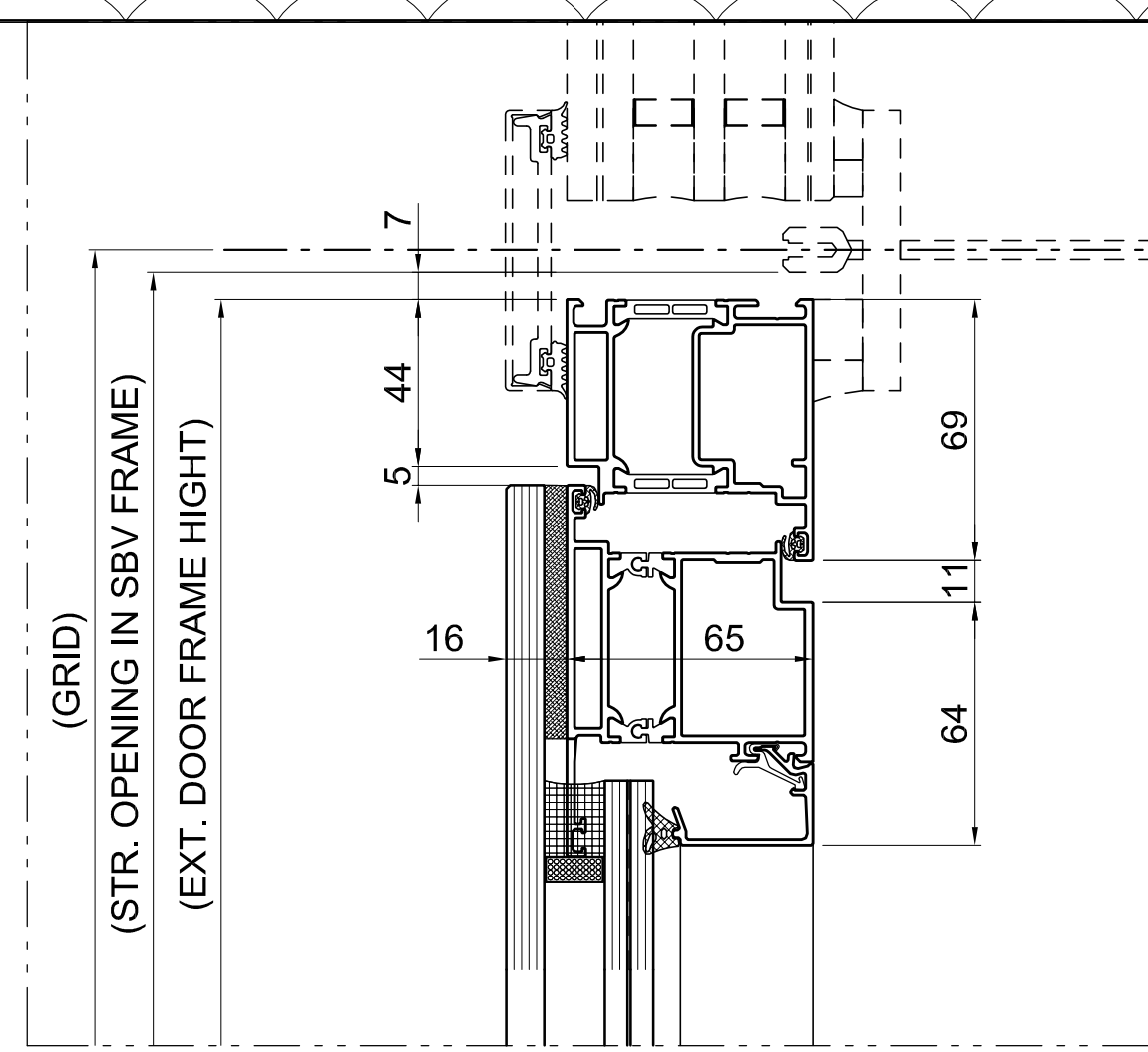
4 VERTICAL SECTION Door type 15 Scale: 1:2
