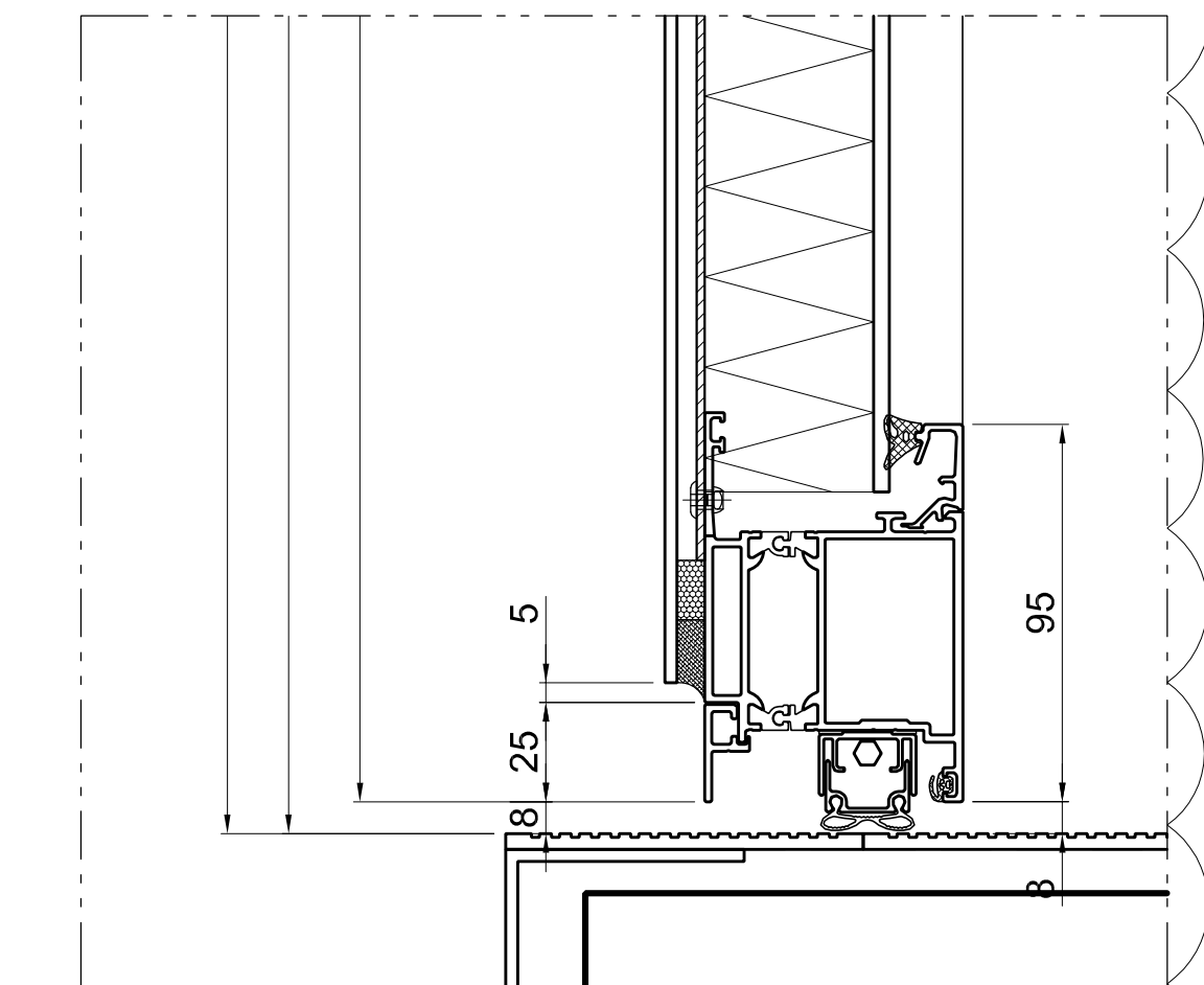
9 VERTICAL SECTION Door type 12 Scale: 1:2
