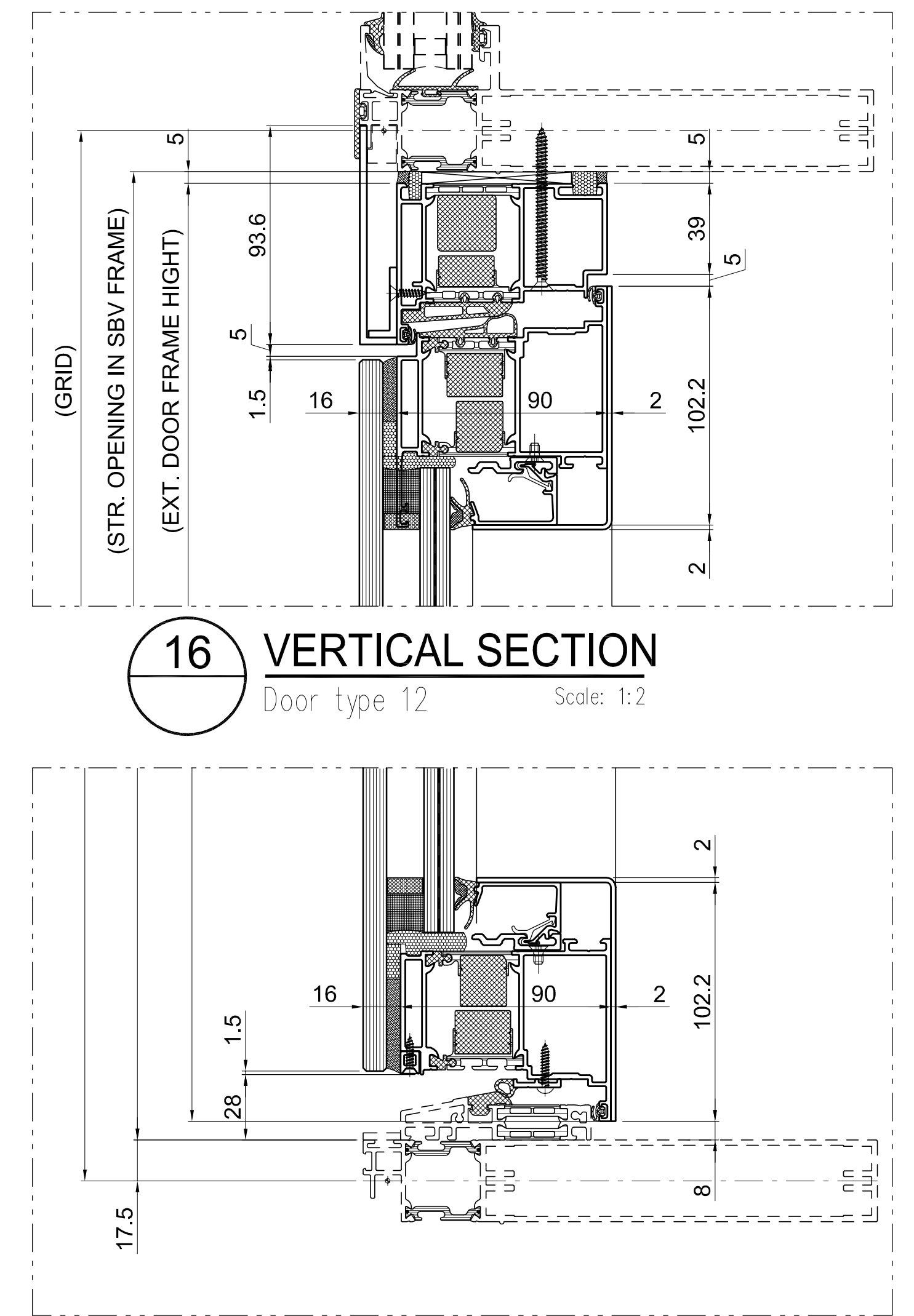
16 VERTICAL SECTION Door type 12 Scale: 1:2
