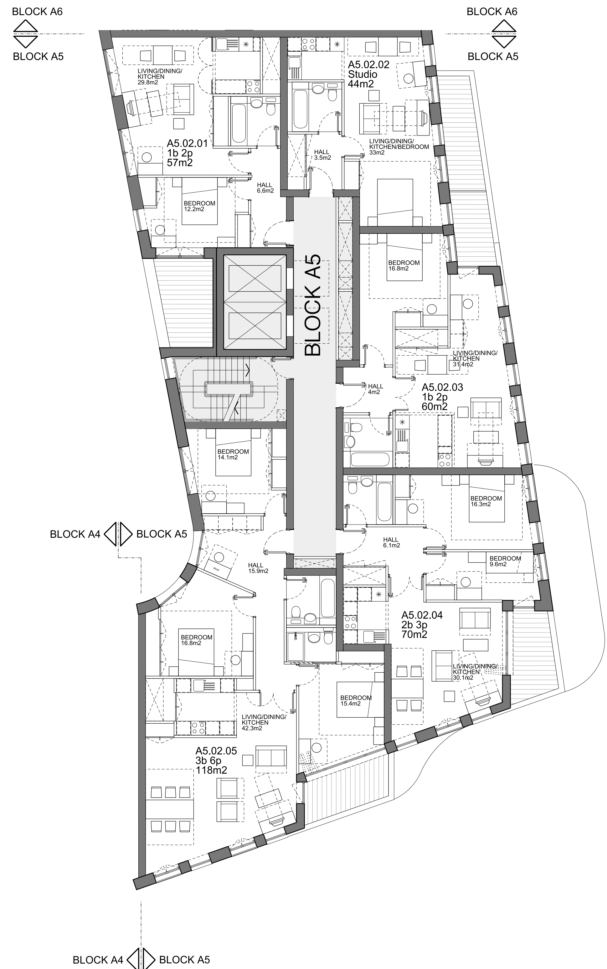
A5 LEVEL 01 +20.45
