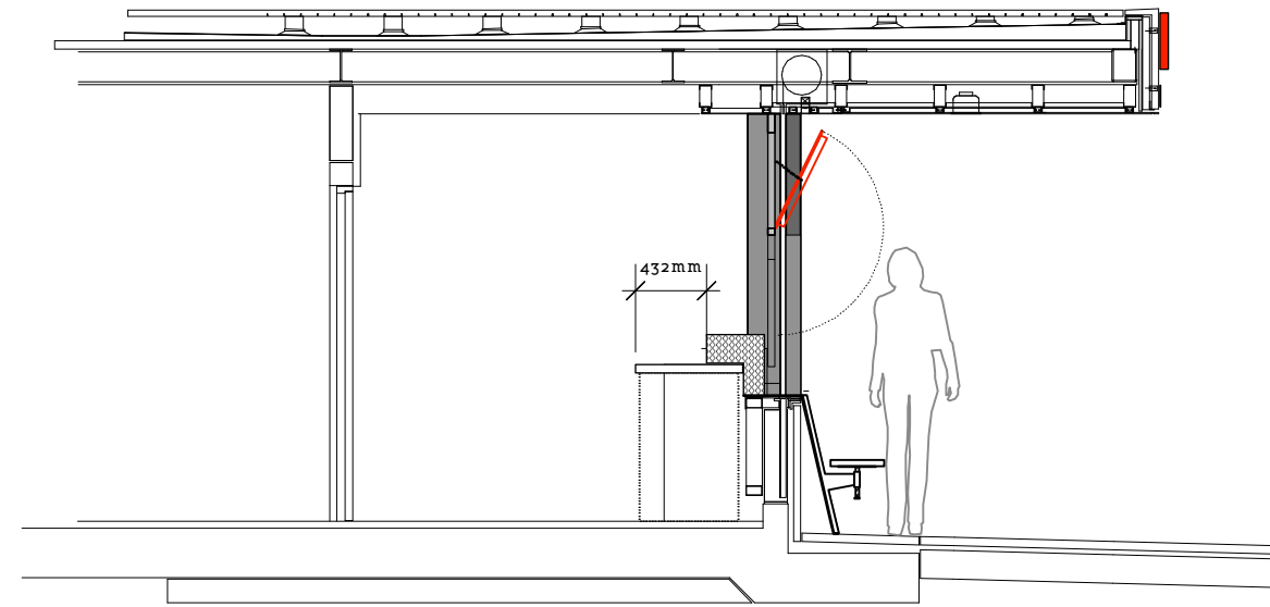
1 SECTION THU. COUNTER SCALE: 1:50
