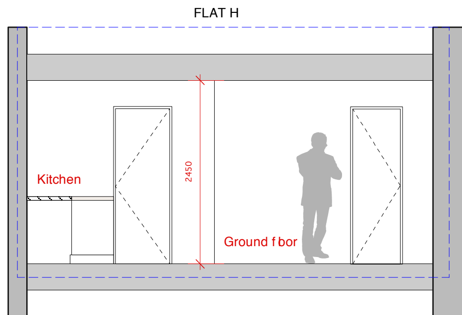
2 Section BB Escale: 1:50@A3
