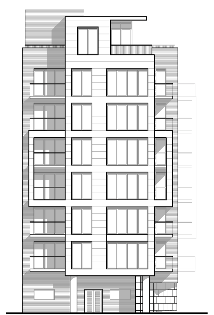
WEST ELEVATION SCALE: 1-200
