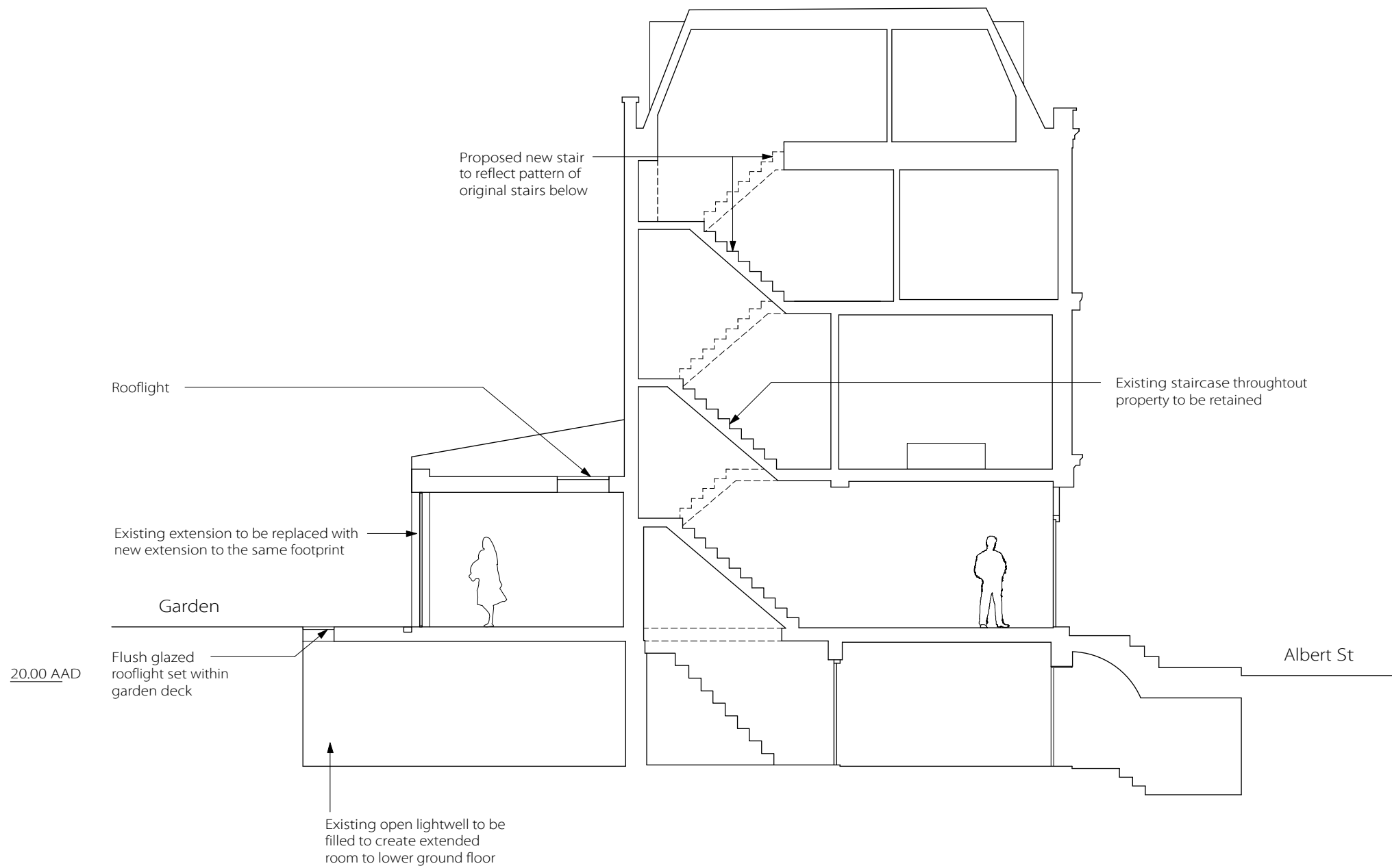
SECTION A-A
