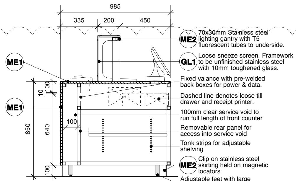
02 SECTION B - TILL 1:20@ A3
