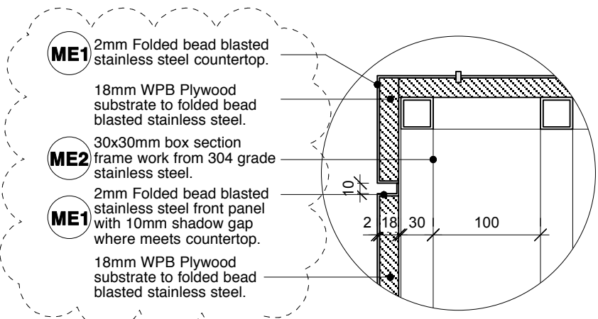
04 DETAIL A 1:5@ A3
